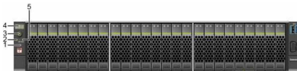
图 3-6 25x2.5 英寸硬盘配置前面板指示灯和按钮
