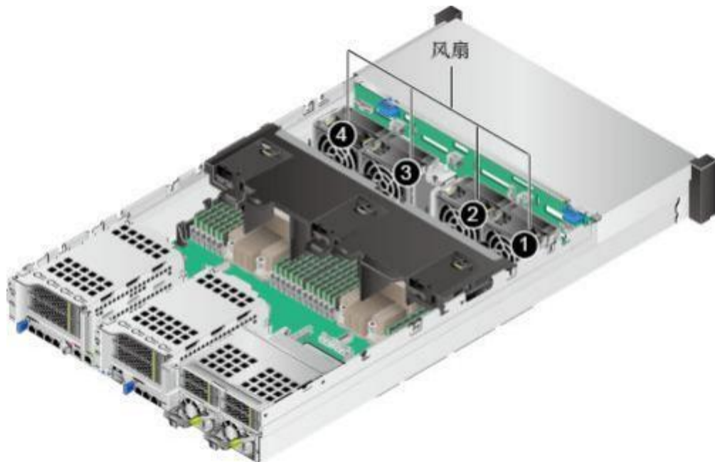
图 3-28 风扇位置图
