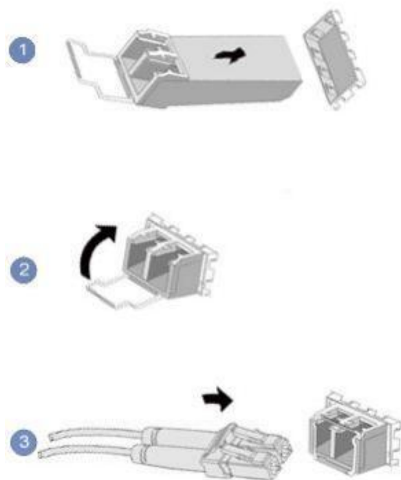
图 6-12 连接光纤
