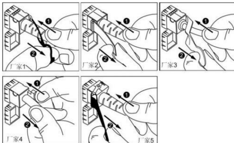
图 6-13 拔出SFP+电缆
