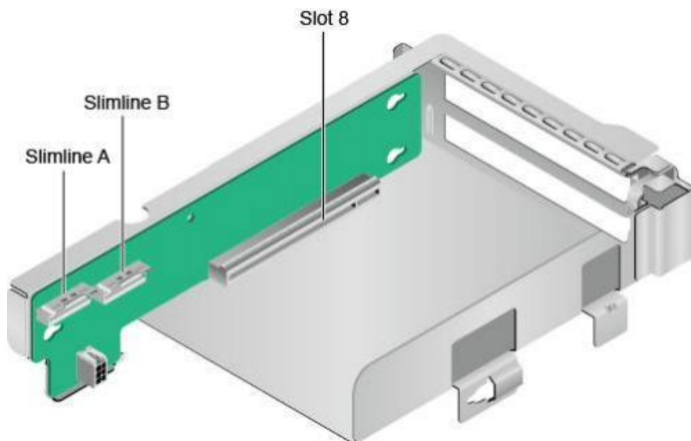
图 3-26 Riser 卡 7 ( 1x16 )
