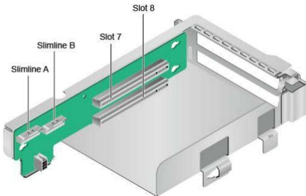
图 3-25 Riser 卡 6 ( 2x8 )
