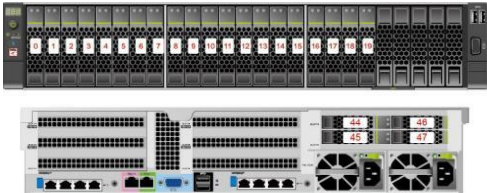
图 3-16 8x2.5 SAS/SATA+12x2.5 NVMe 硬盘配置硬盘编号
