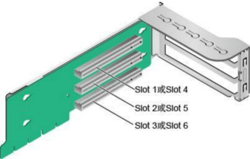
图 3-20 Riser 卡 1（3x8）
