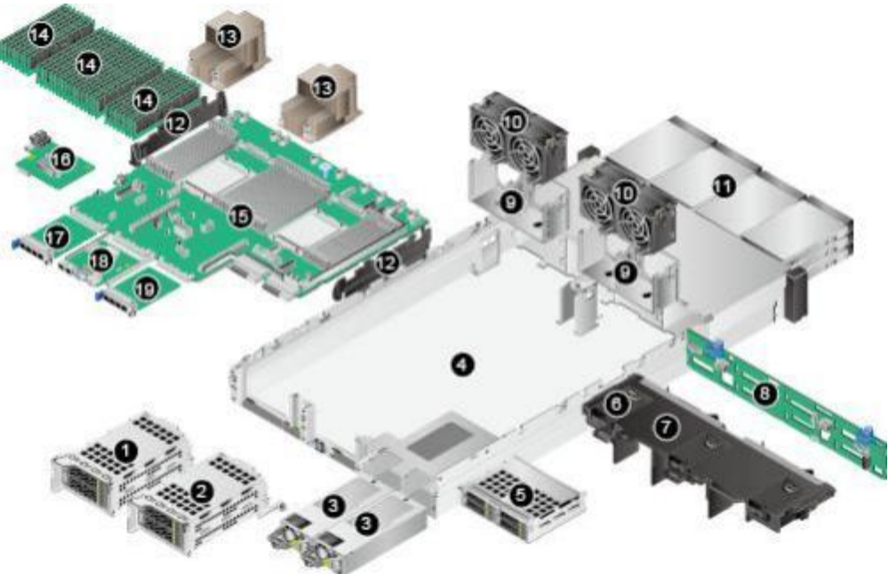
图 2-2 部件
