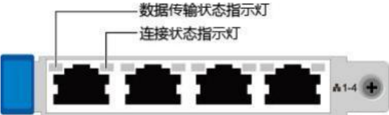
图 3-11 TM210（4*GE 电口）
