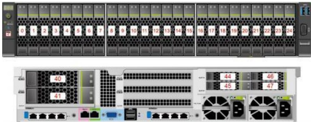
图 3-15 25x2.5 英寸硬盘 EXP 配置硬盘编号
