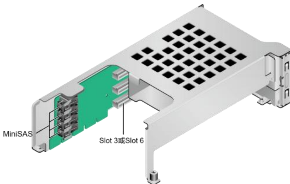
图 3-24 Riser 卡 5 ( SAS Riser)
