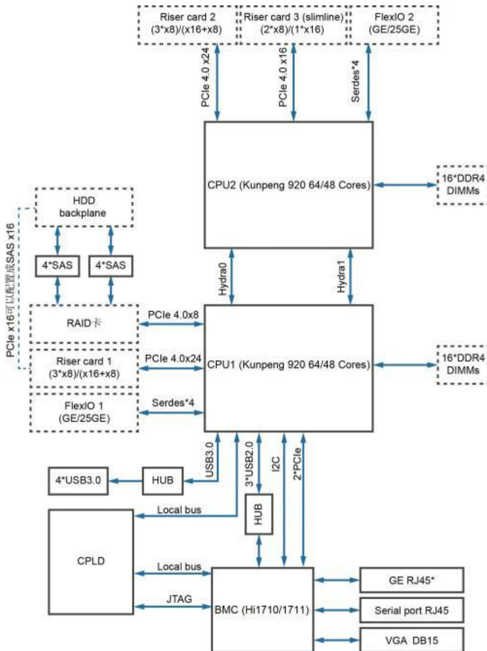
图 2-3 擎天 RK6260 V5服务器 逻辑结构
