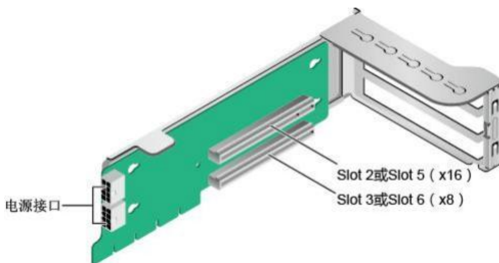
图 3-21 Riser 卡 2 (1x8+1x16)
