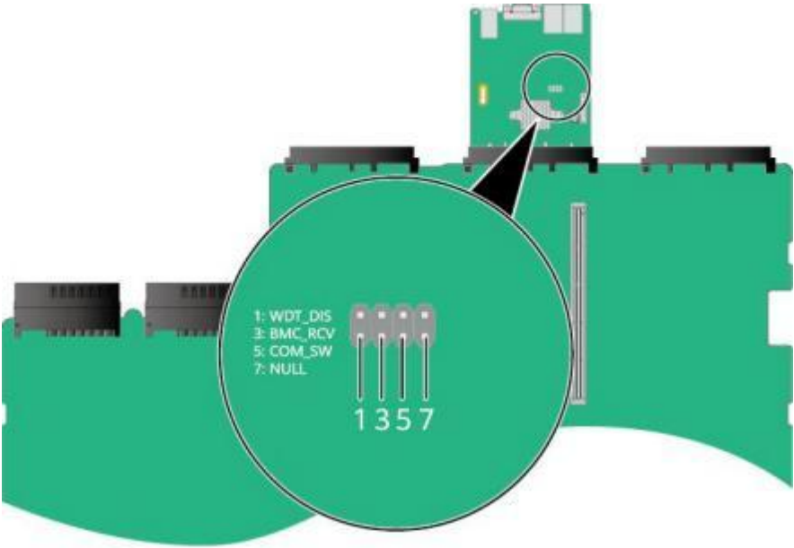
图 8-13 跳线位置
