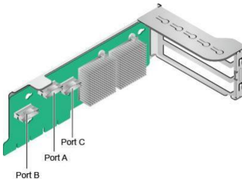
图 3-22 Riser 卡 3 ( 12NVMe 专用 )
