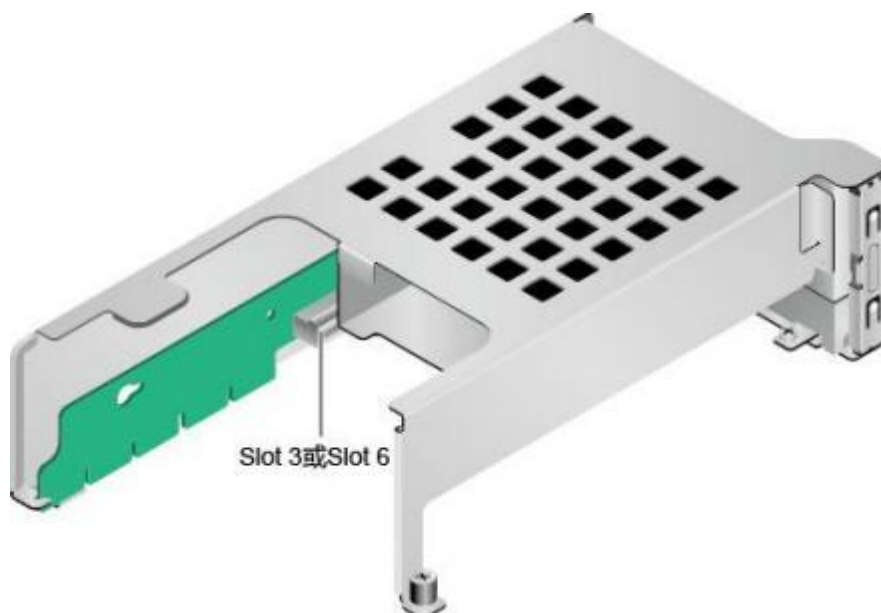
图 3-23 Riser 卡 4 ( 1x16 )
