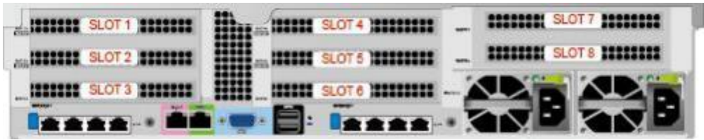
图 3-27 PCIe 插槽
