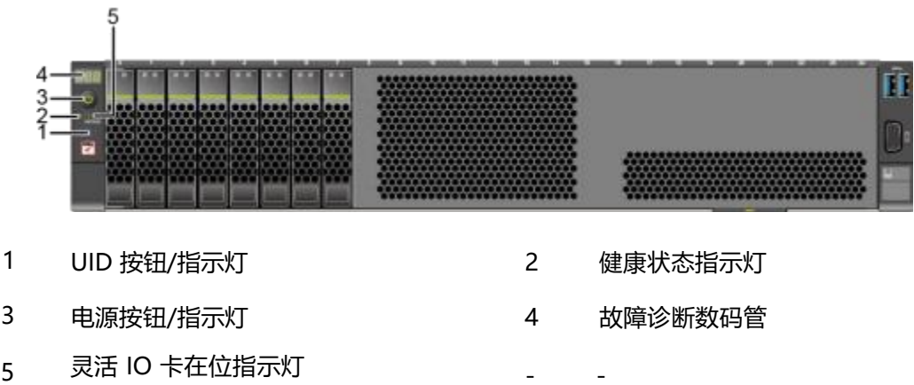
图 3-8 8x2.5 英寸硬盘配置前面板指示灯和按钮
