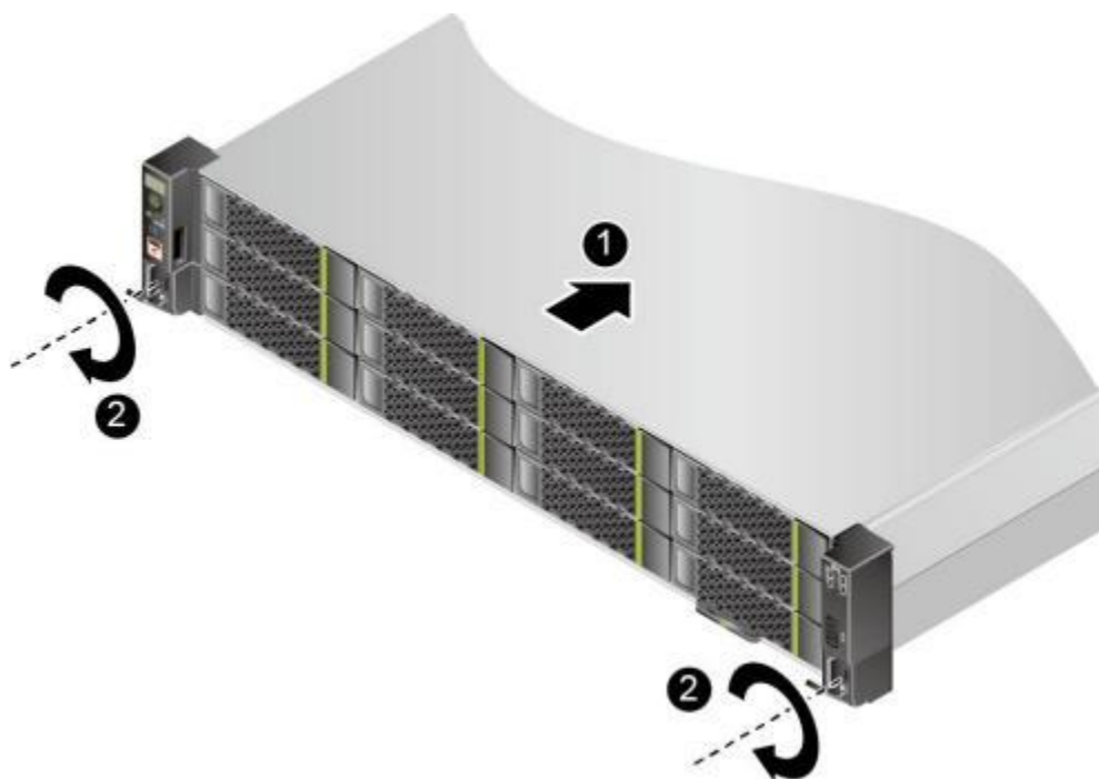
图 6-9 安装服务器
