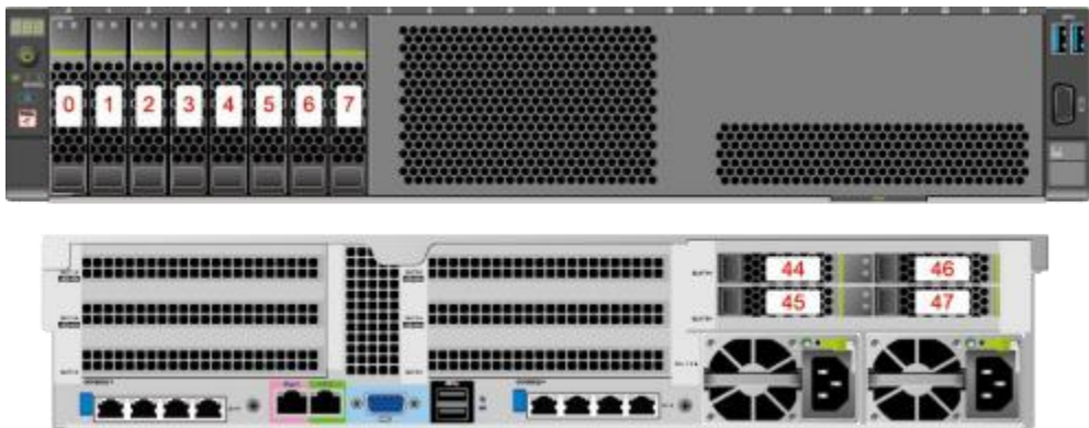
图 3-17 8x2.5 英寸硬盘配置的硬盘编号
