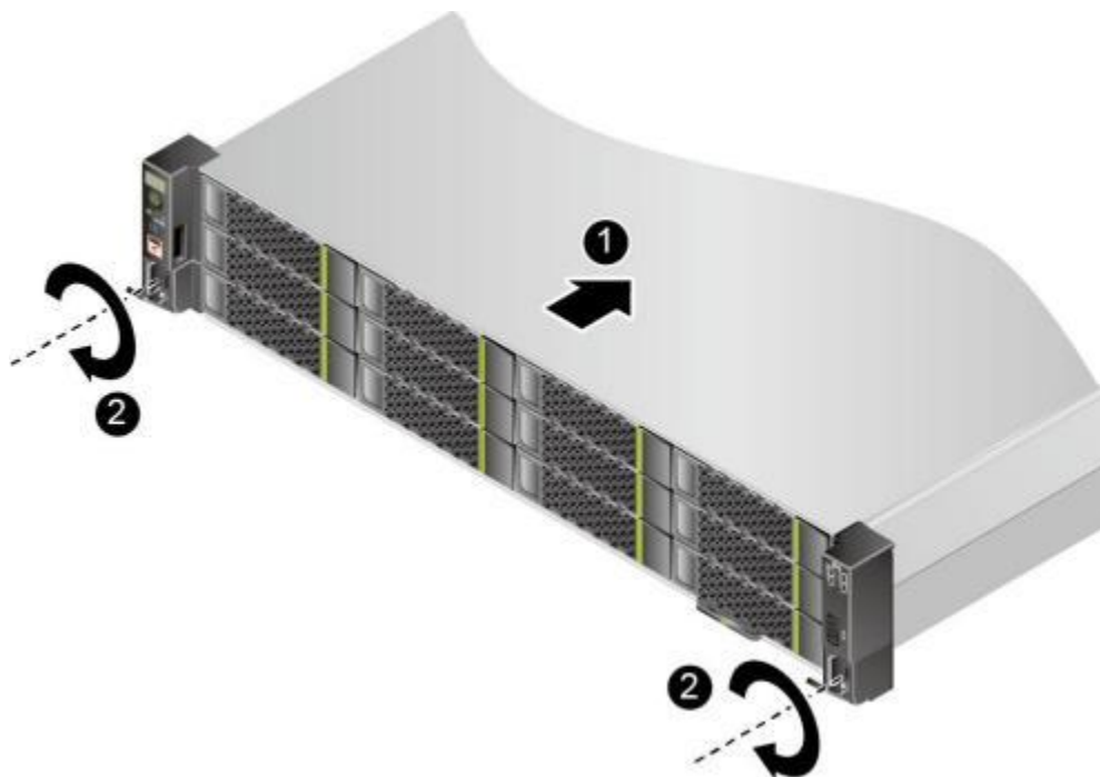
图 6-7 安装服务器
