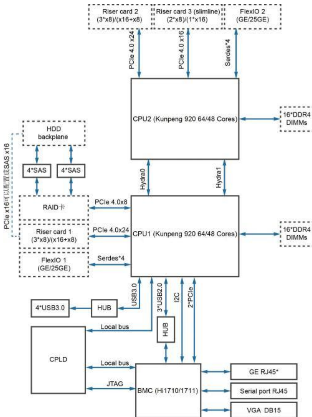
图 2-3 擎天 RK5260 V5服务器 逻辑结构
