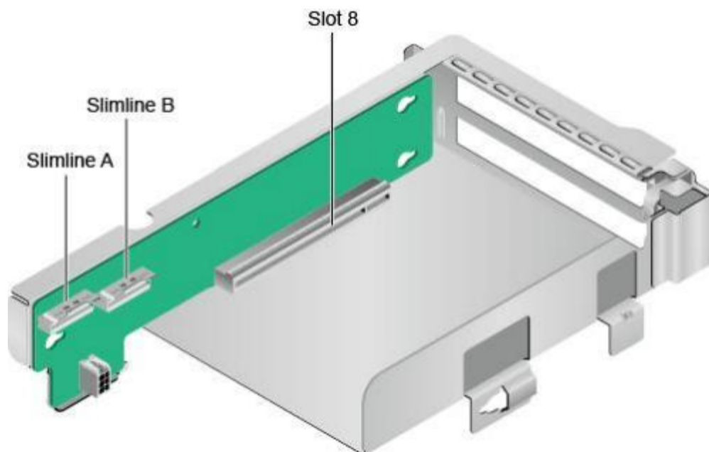
图 3-26 Riser 卡 7 ( 1x16 )
