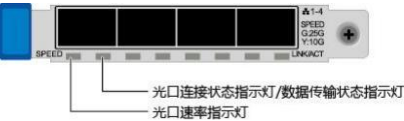
图 3-12 TM280 (4*25GE 光口 )
