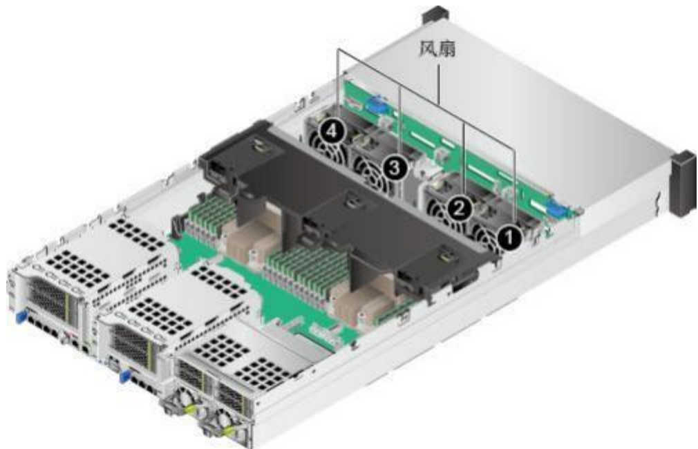
图 3-28 风扇位置图
