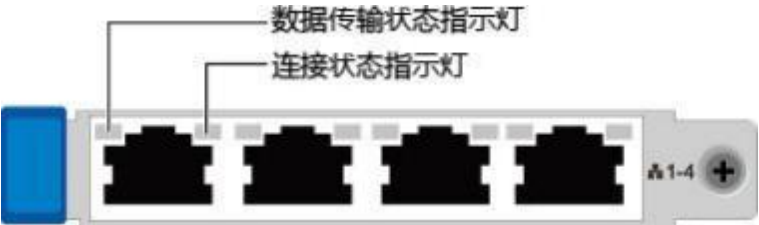
图 3-11 TM210（4*GE 电口）
