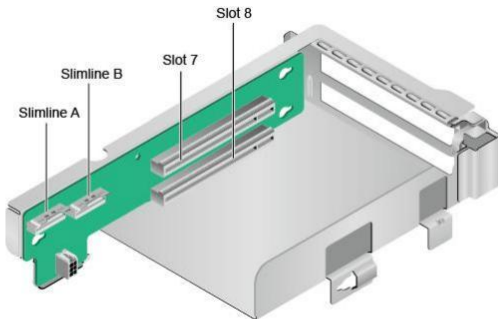
图 3-25 Riser 卡 6 ( 2x8 )
