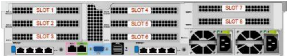
图 3-27 PCIe 插槽
