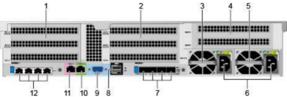
图 3-9 后面板组件
