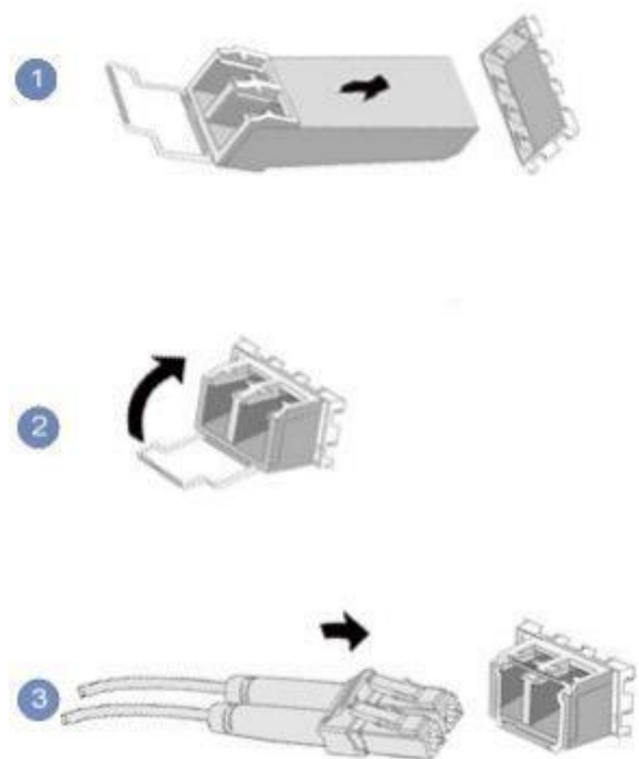
图 6-12 连接光纤
