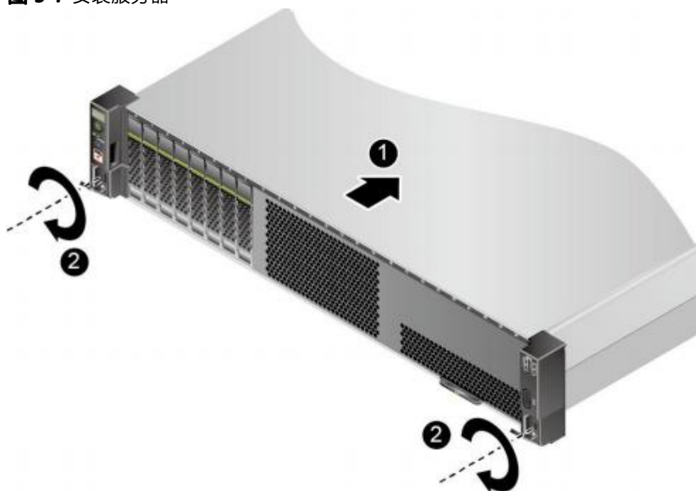
图 5-7 安装服务器
