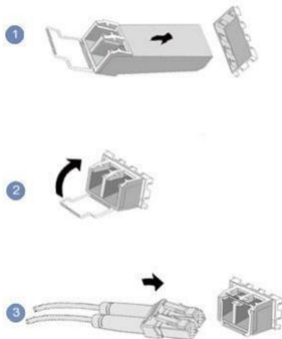
图 5-12 连接光纤
