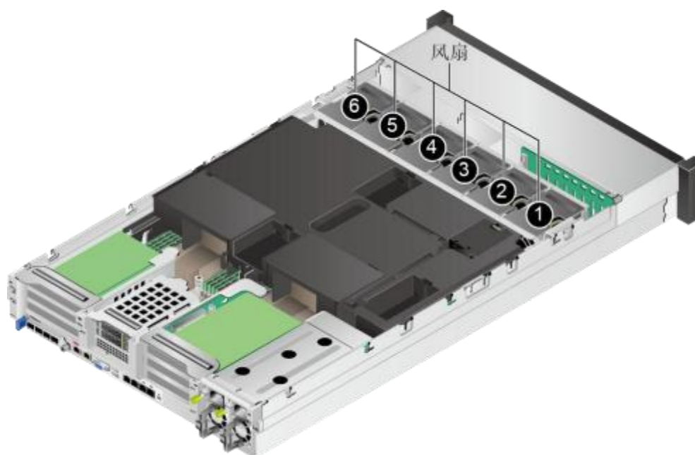
图 2-15 风扇位置图
