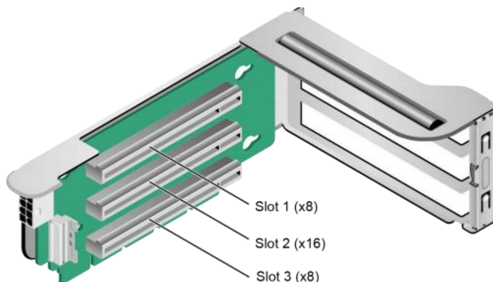
图 2-12 Riser 卡1
