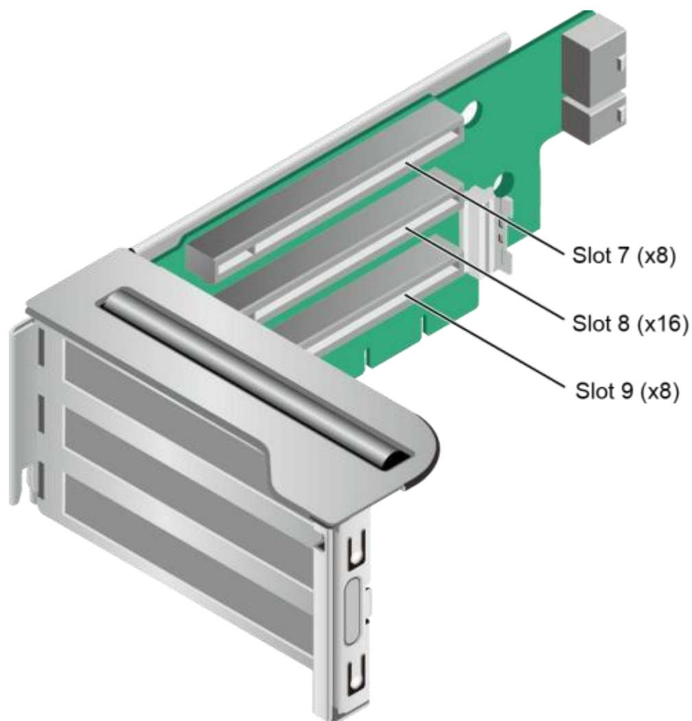
图 2-14 PCIe 插槽
