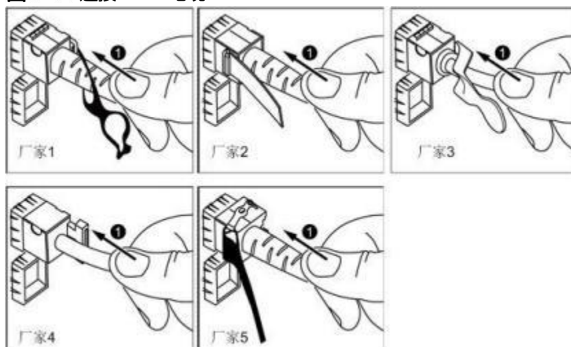
图 5-14 连接 SFP+ 电缆
