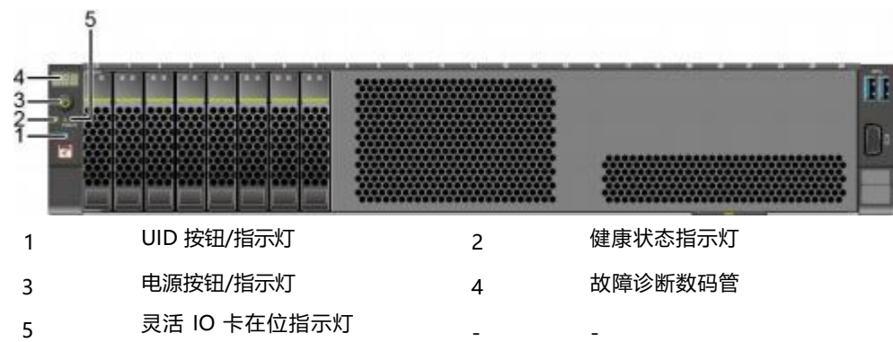
图 2-4 8x2.5 英寸硬盘配置前面板指示灯和按钮
