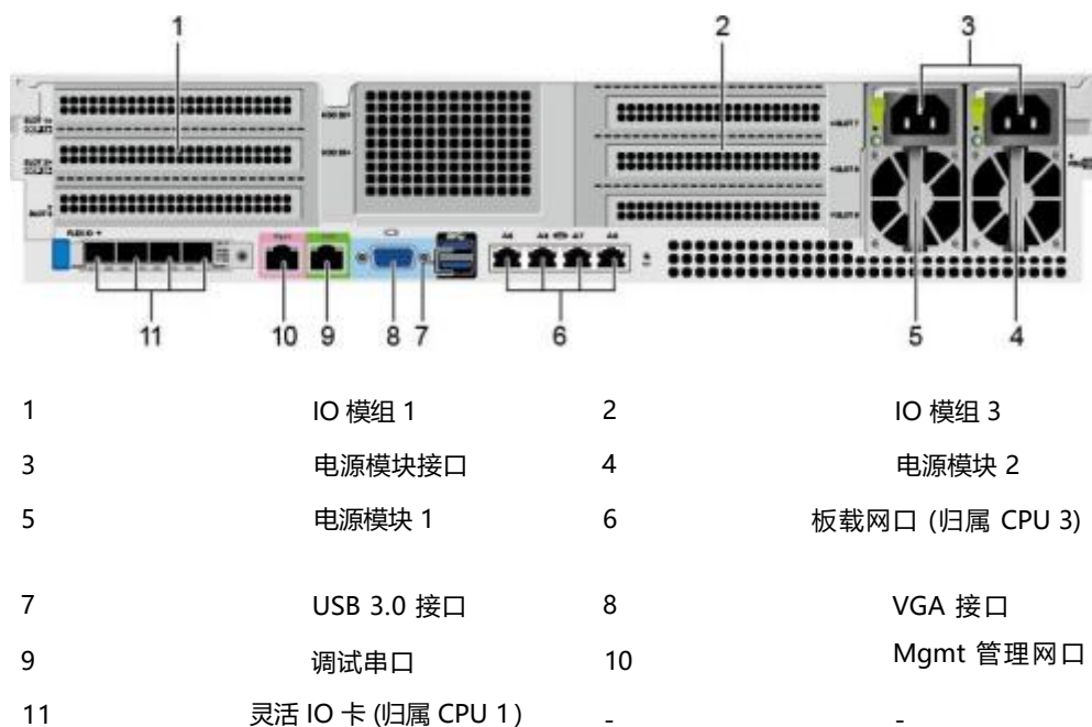
图 2-6 后面板组件
