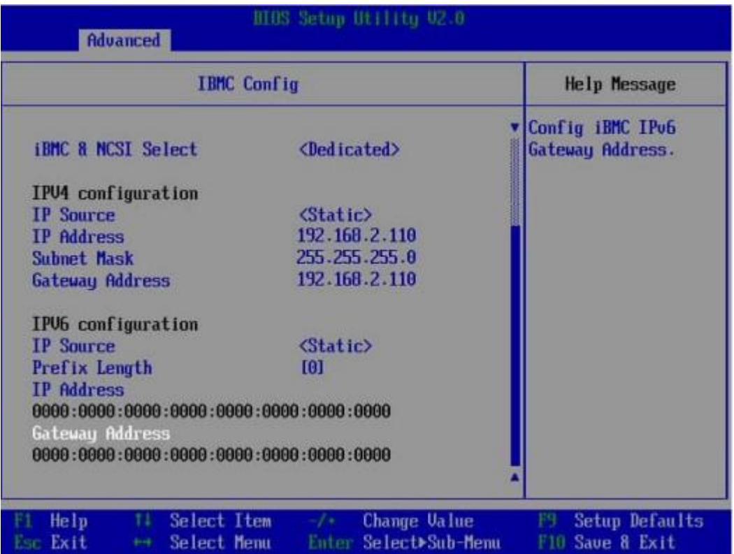
图 5-22 IBMC Config 界面2
