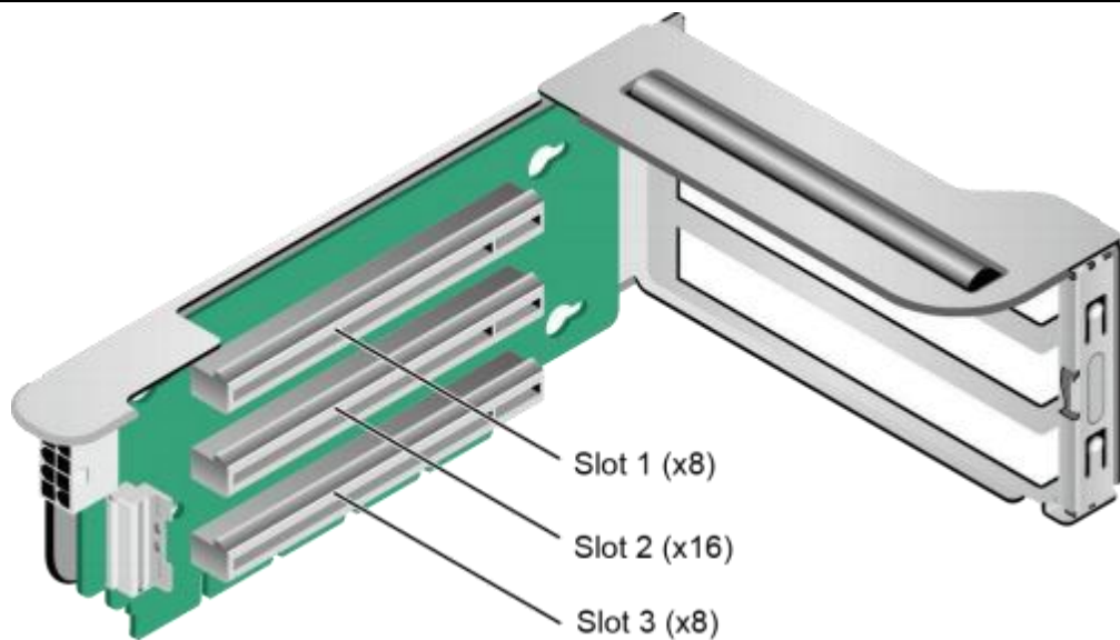
图 4-11 Riser 卡 2
