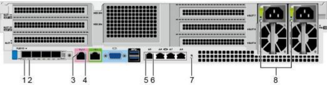
图 4-7 后面板指示灯
