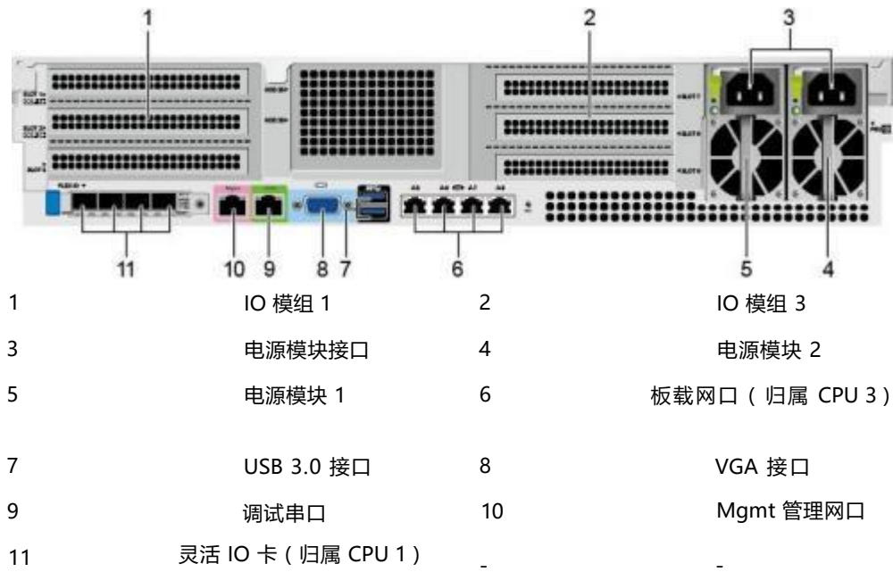
图 4-4 后面板组件
