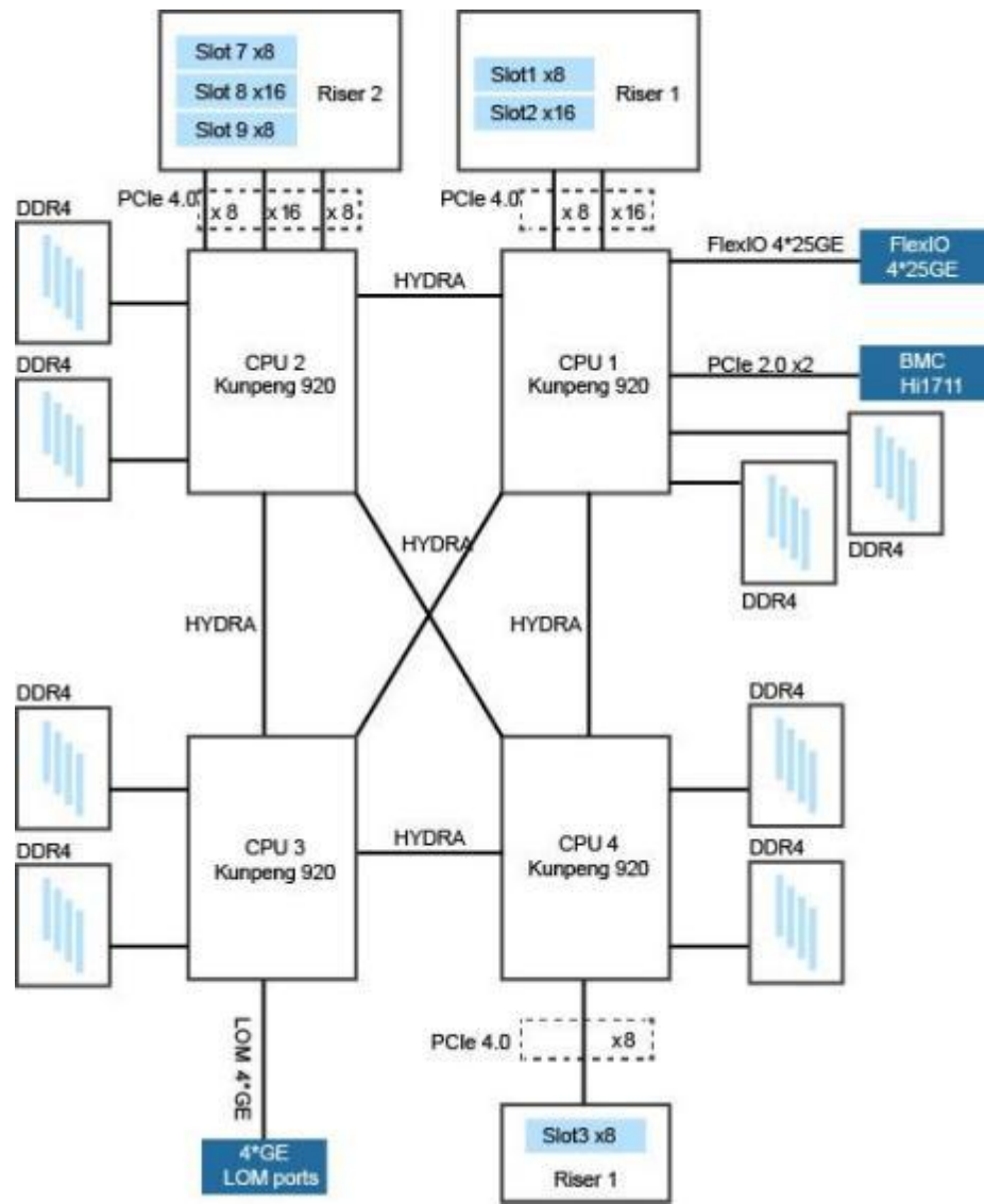
图 3-1 擎天 RK7460 V5 逻辑结构
