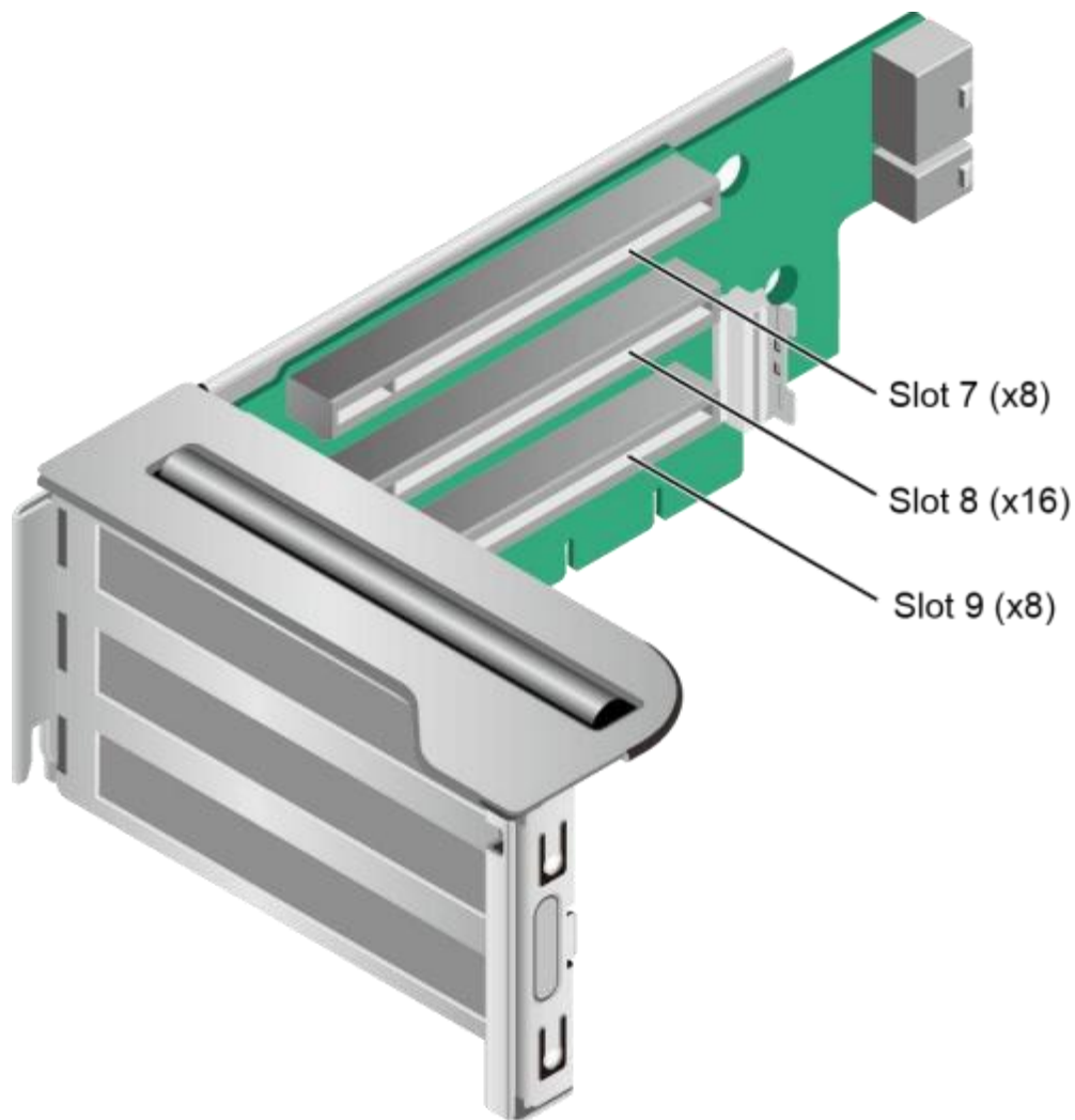
图 4-11 Riser 卡 2
