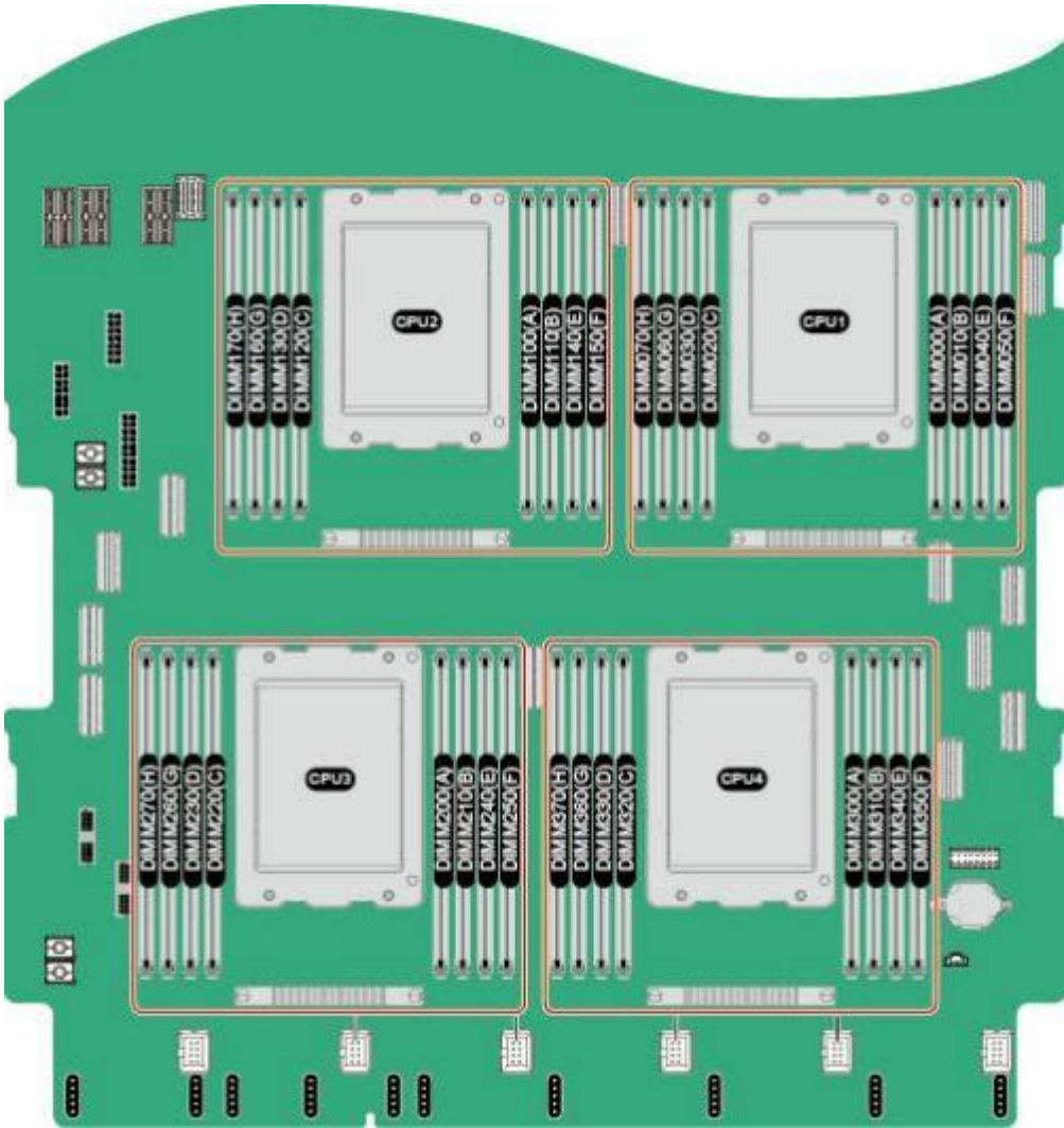
图 6-1 DIMM 安装位置
