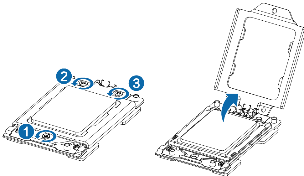
图 2-7 打开 Force Frame 示意图
