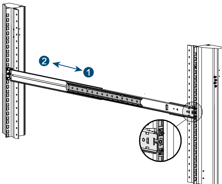
图 2-22 安装外导轨到机柜立柱示意图
