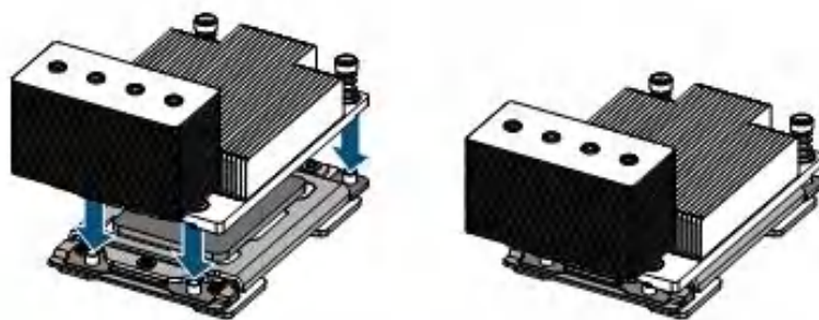
图 2-10 安装散热器示意图
