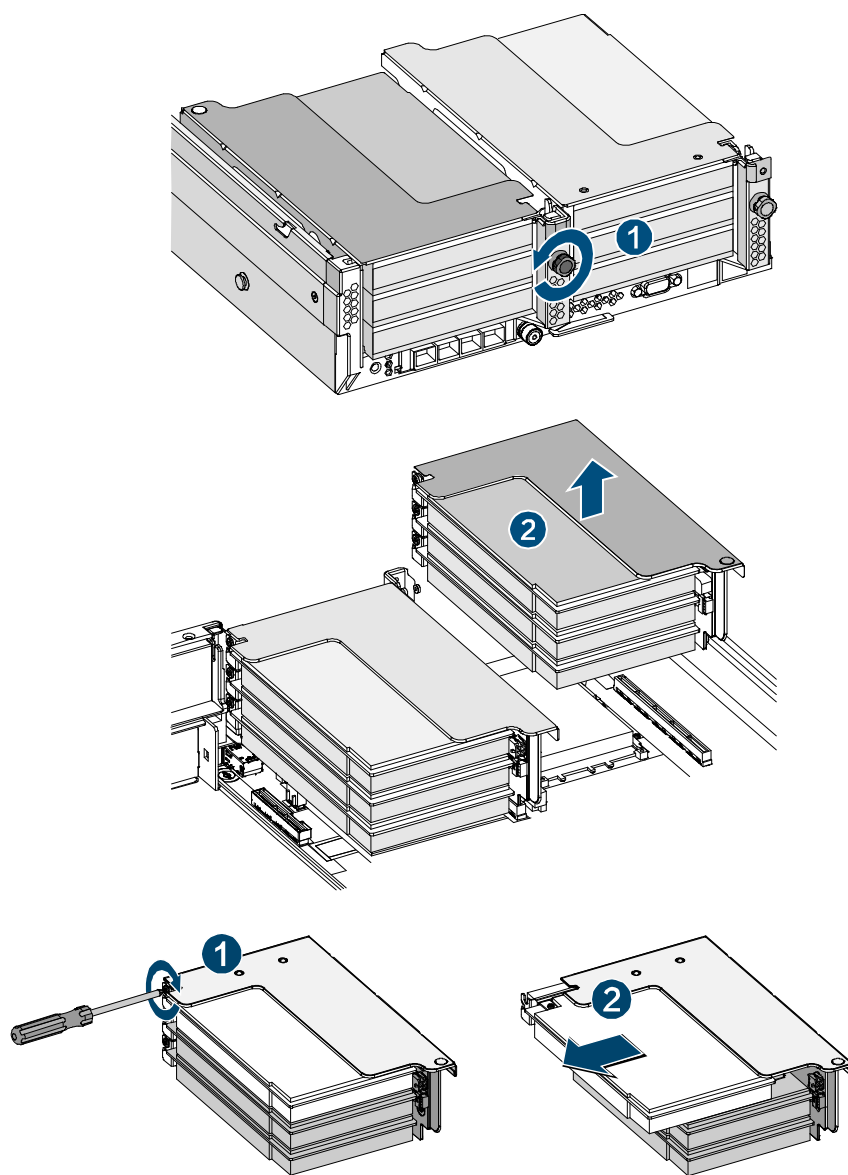
图 2-16 机箱扩展卡安装示意图
