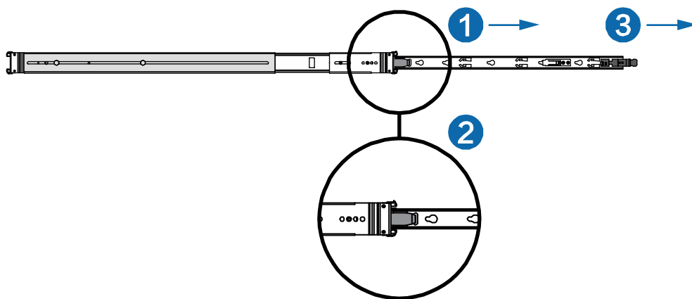
图 2-20 抽出内轨示意图
