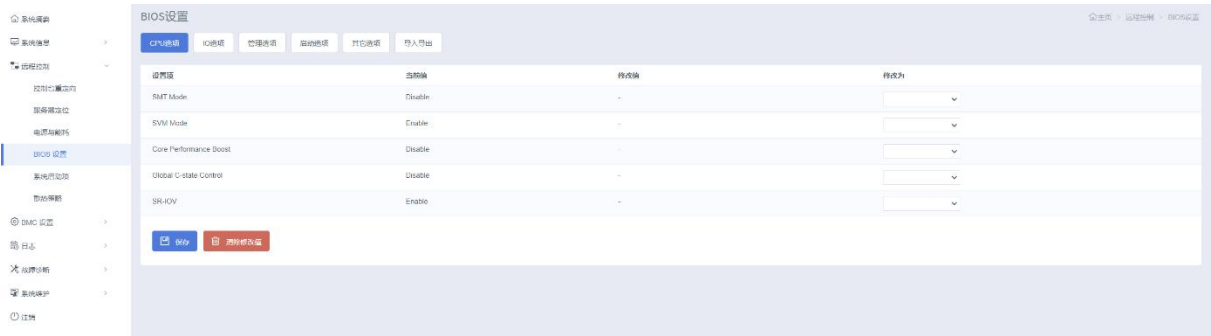
图 3-81 BIOS 设置
