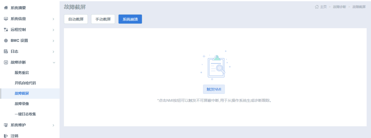
图 3-112 系统崩溃图
