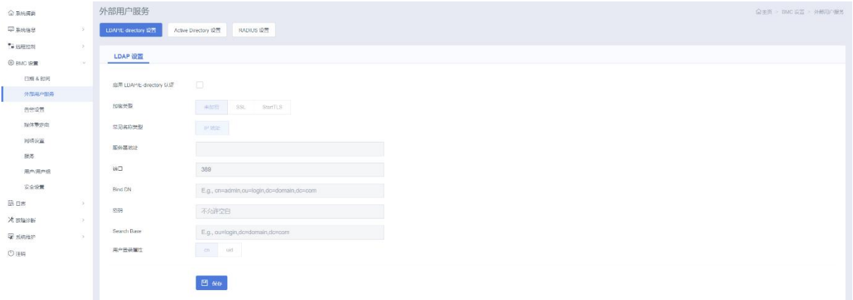
图 3-87 LDAP/E-directory 设置
