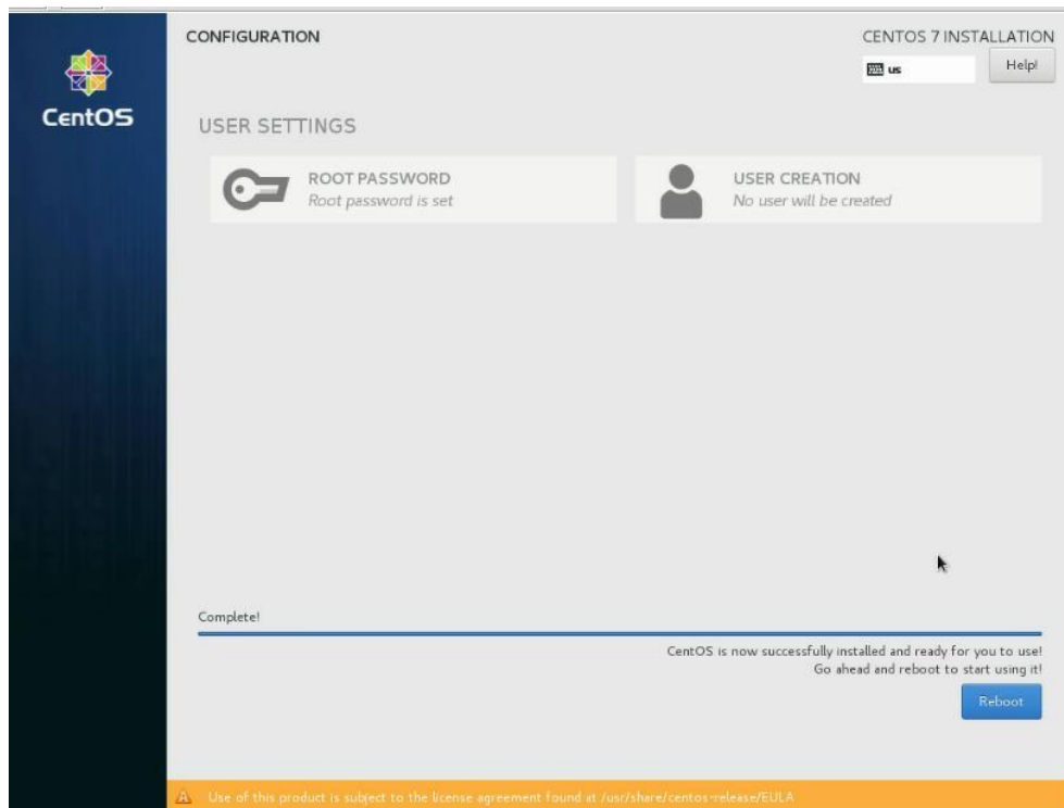
图 4-32 安装完成
