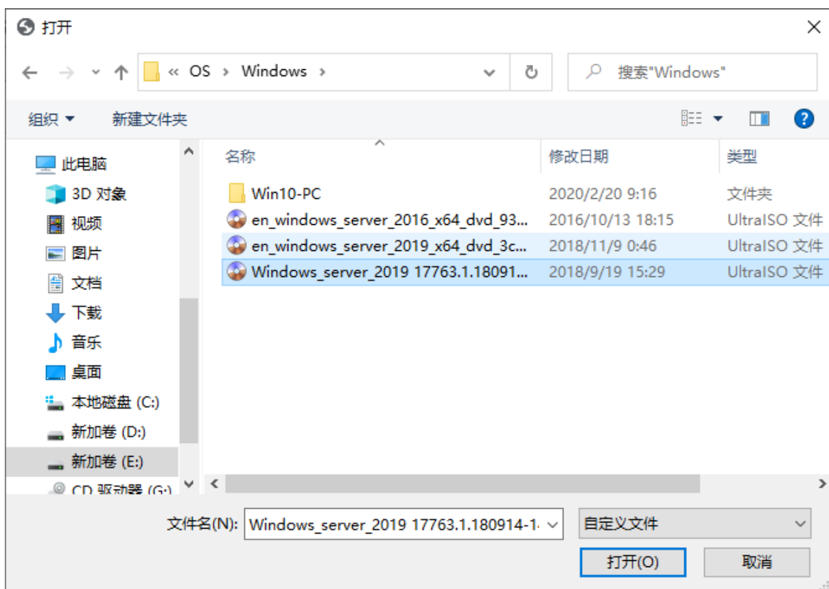
图 4-5 挂载界面
