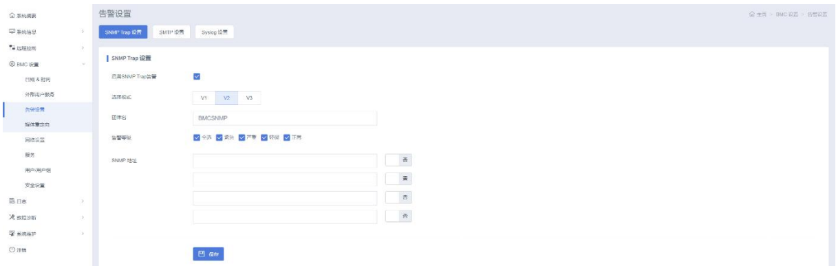
图 3-90 告警设置
