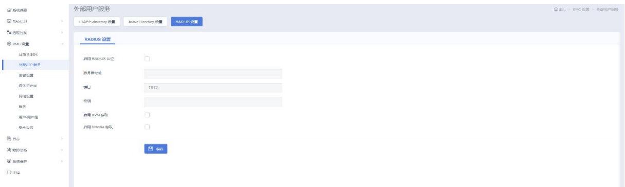
图 3-89 RADIUS 设置
