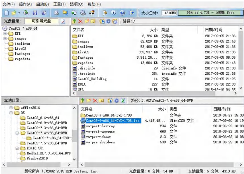
图 4-34 UltraISO 界面
