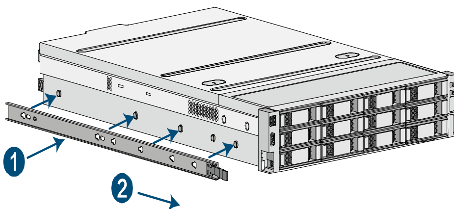
图 2-21 安装内轨示意图
