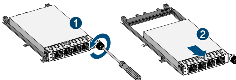
图 2-18 OCP 卡拔出示意图
