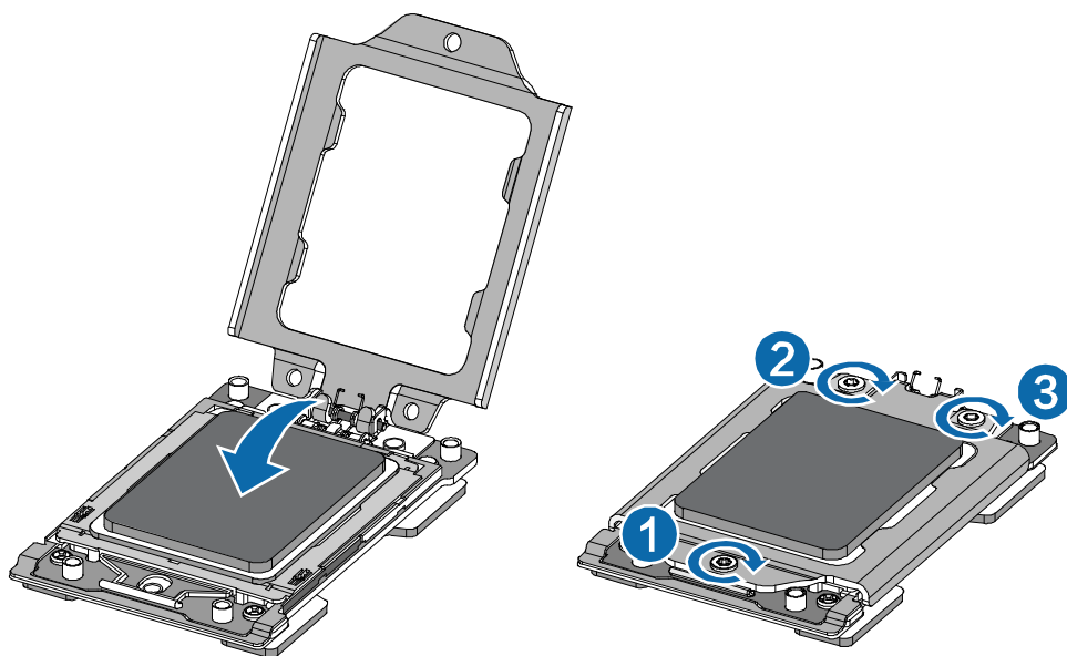
图 2-9 安装 CPU 示意图
