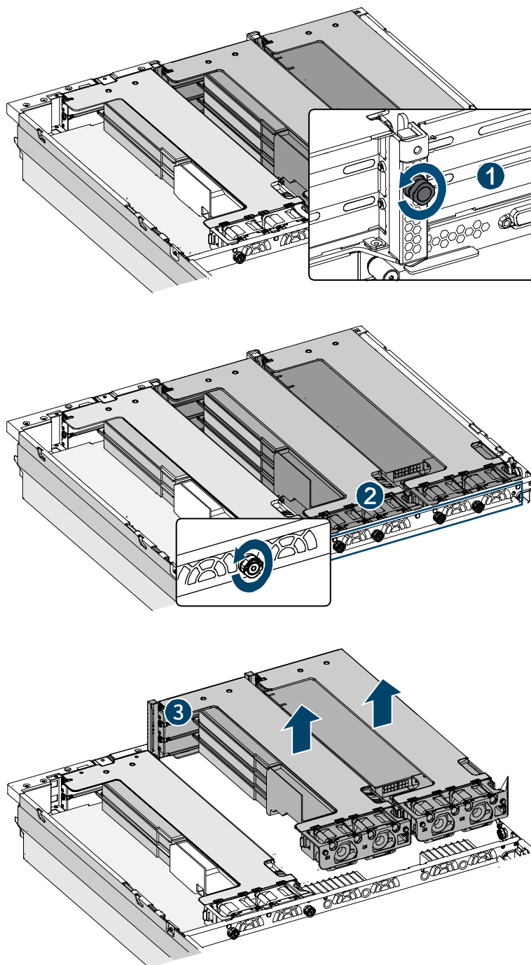
图 2-15 GPU 卡拆装示意图
