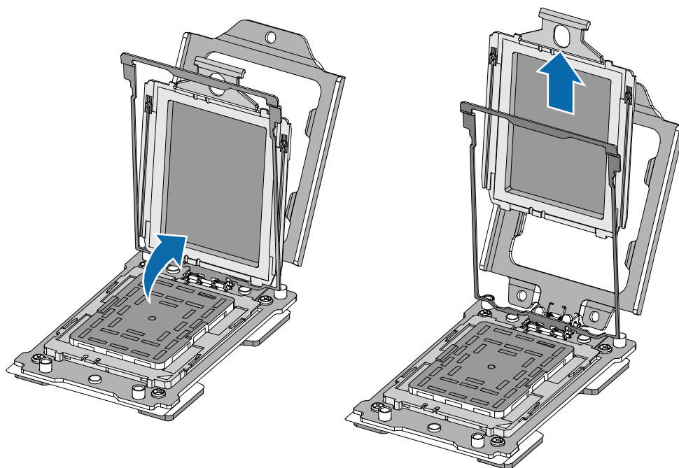
图 2-8 拔出 External Cap 示意图
