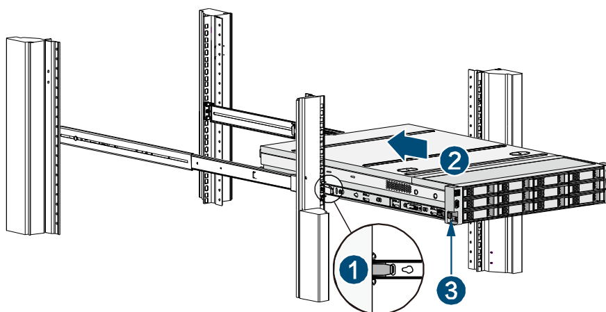
图 2-23 将机器安装到外轨示意图
