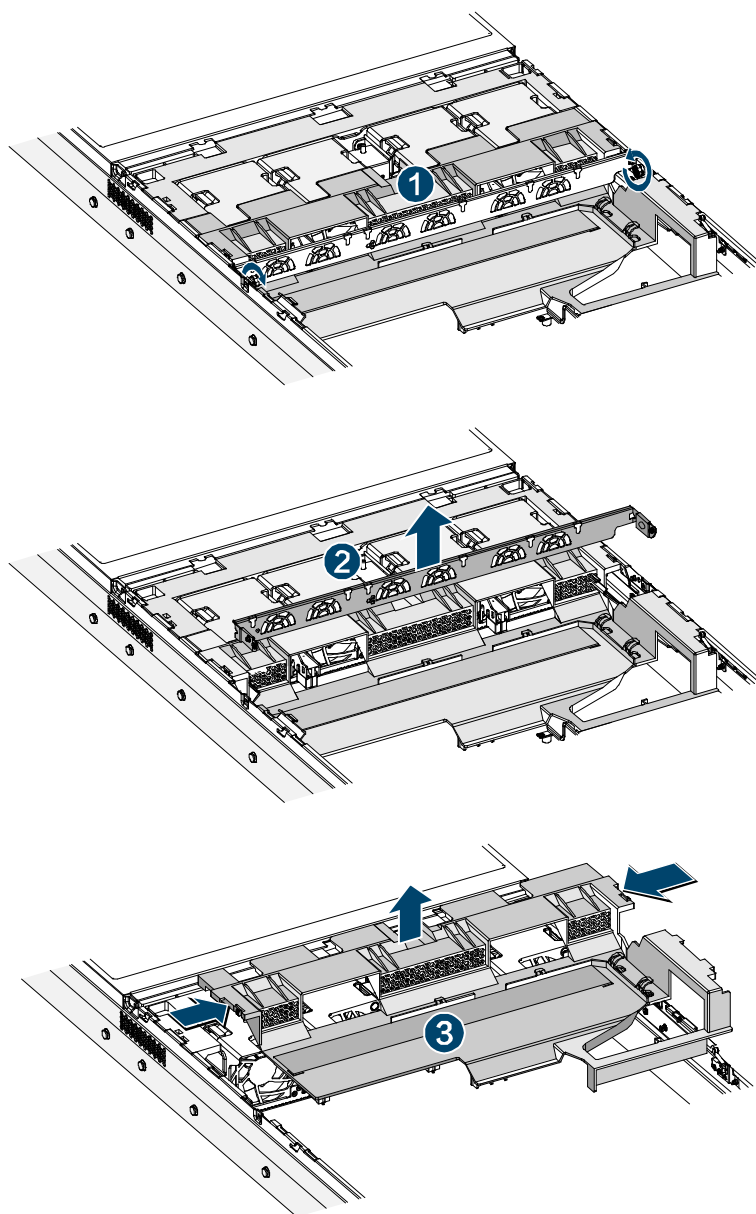
图 2-6 取 GPU 支架和导风罩示意图
