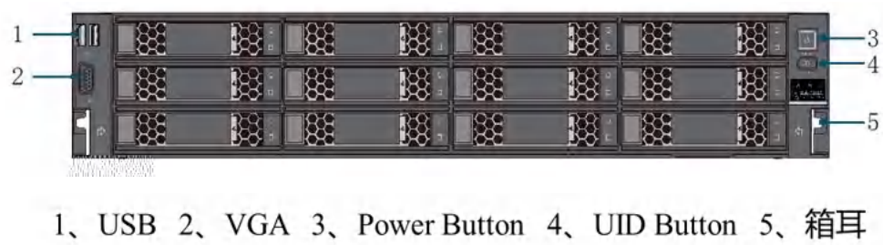
图 2-1 前面板示意图
