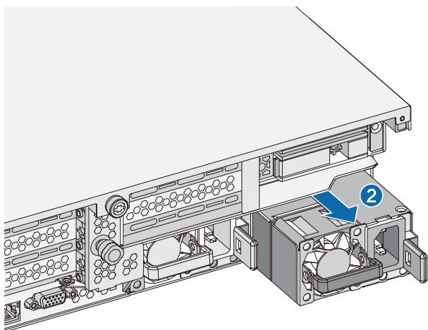
图 2-14 拔出电源模块示意图
