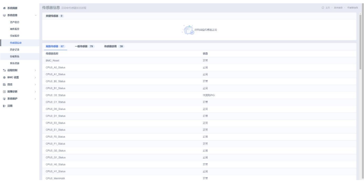
图 3-66 传感器读数
