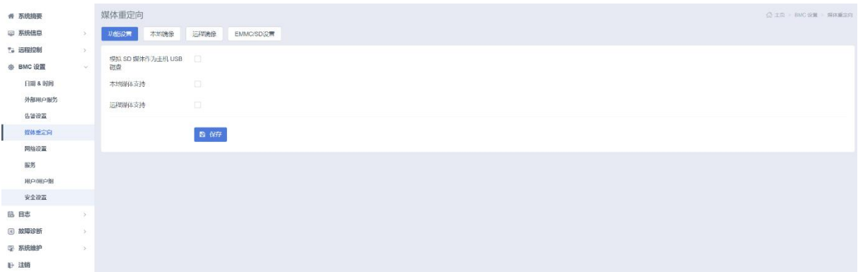
图 3-91 媒体重定向
