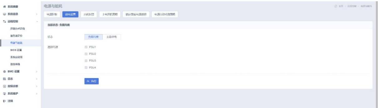
图 3-76 供电设置
