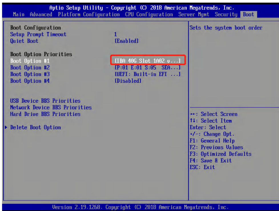
图 4-39 启动项设置
