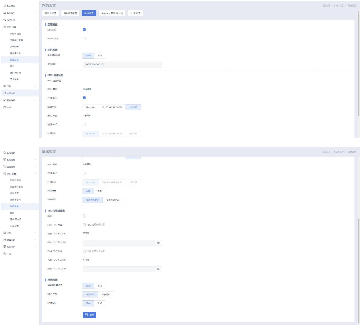
图 3-95 DNS 配置
