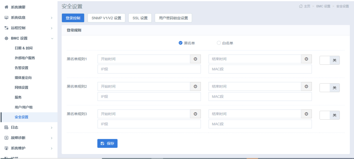
图 3-100 登陆控制
