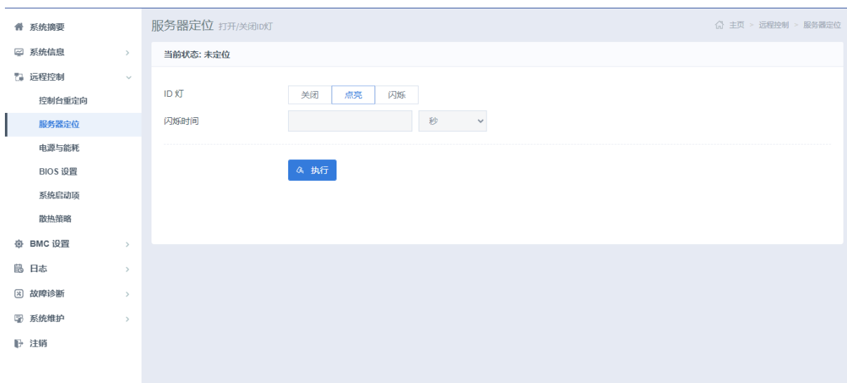
图 3-73 服务器定位
