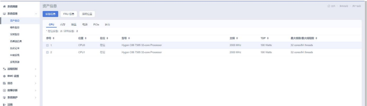
图 3-63 资产信息图
