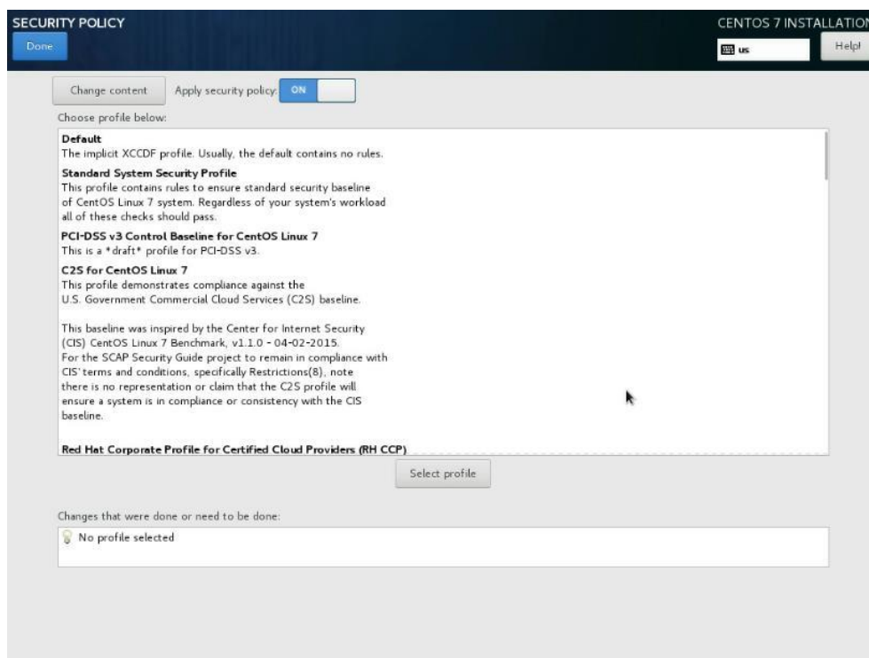
图 4-29 安全策略
