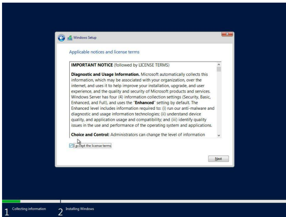
图 4-11 许可条款
