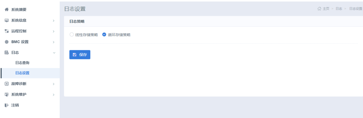
图 3-107 日志设置
