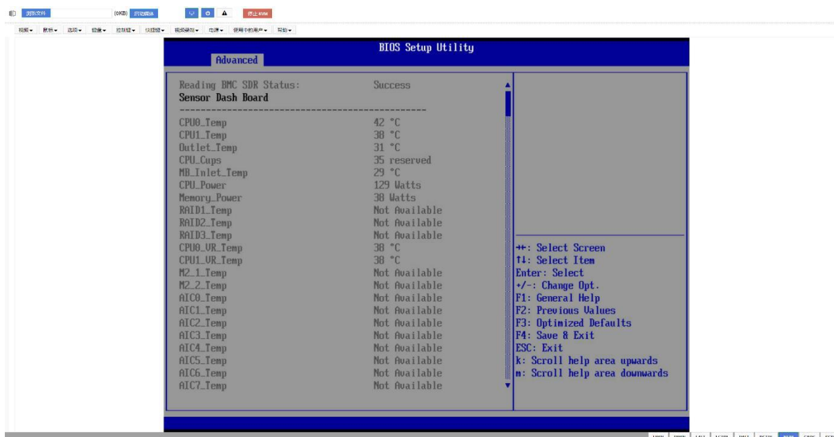
图 3-72 H5 KVM
