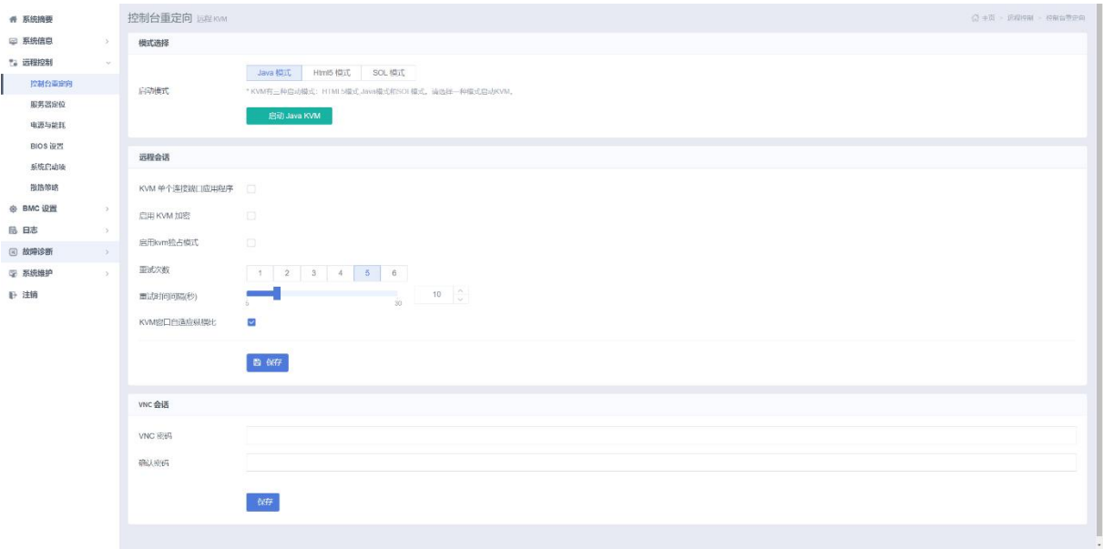
图 3-69 远程控制
