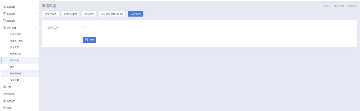
图 3-97 LLDP 设置
