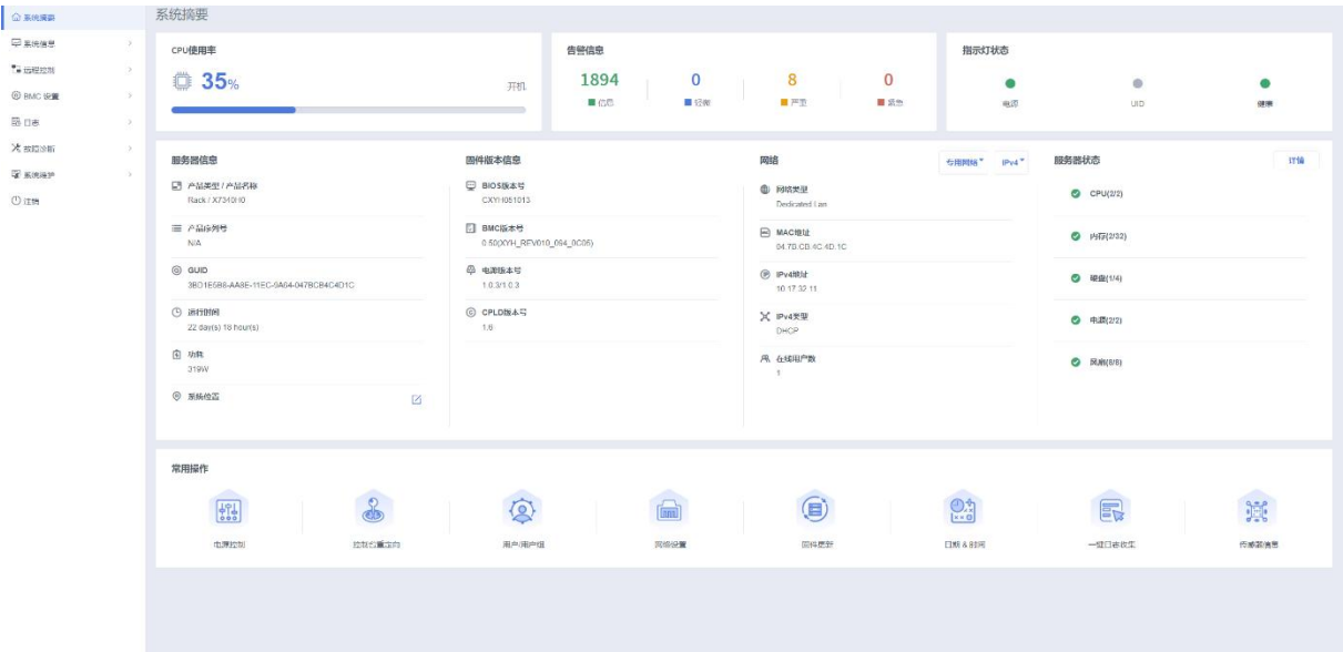
图 3-61 BMC 主界面
