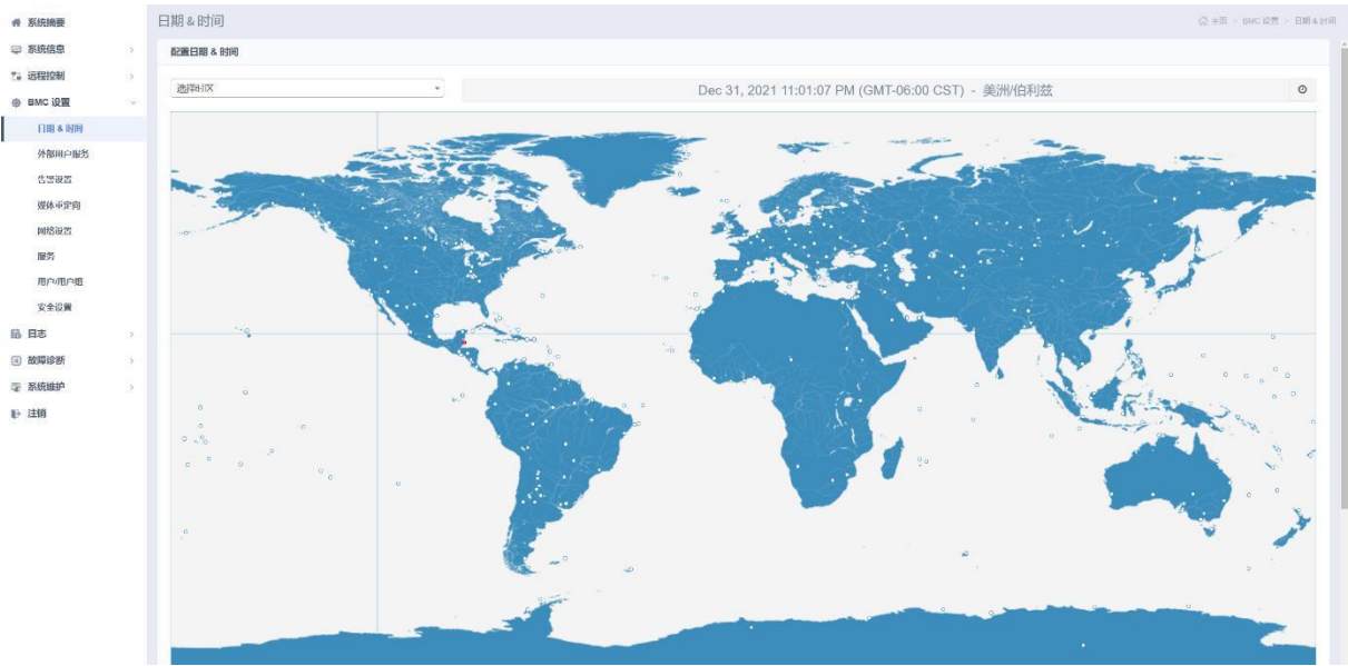
图 3-84 BMC 设置
