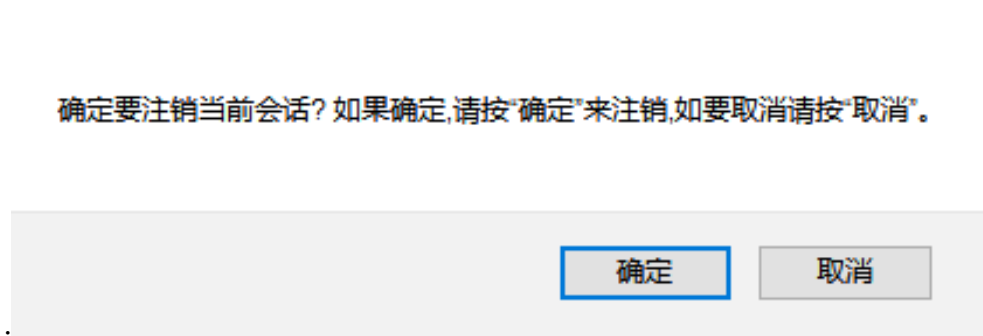
图 3-121 注销对话框
