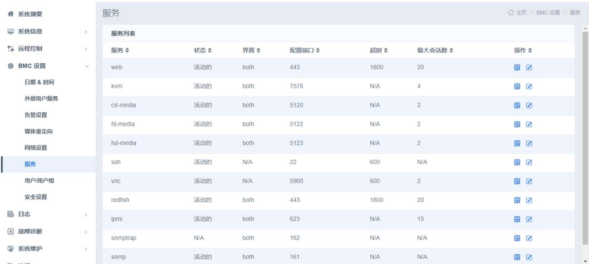
图 3-98 服务设置
