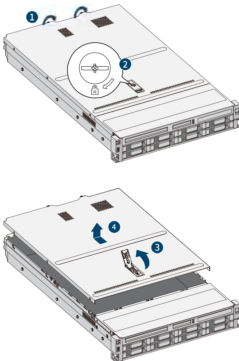
图 2-5 开启机箱盖示意图
