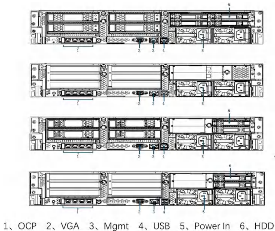
图 2-4 产品后视图
