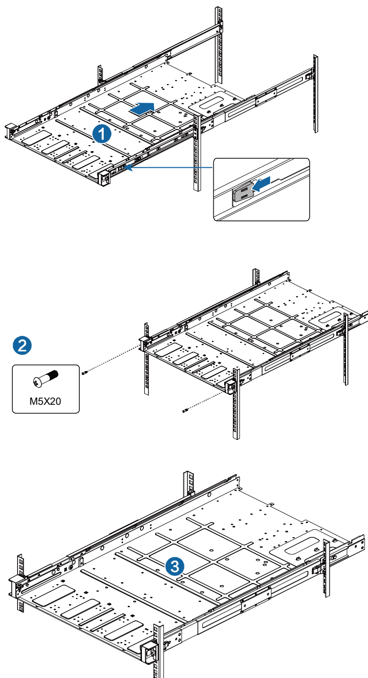
图 2-21 机箱锁定示意图
