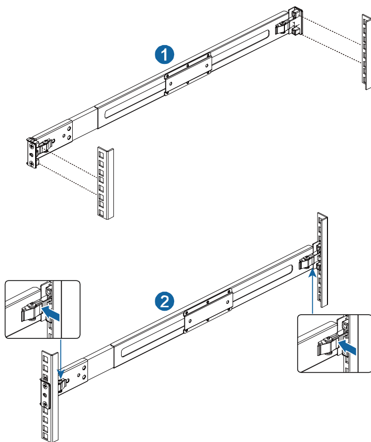
图 2-19 安装外导轨到机柜立柱示意图
