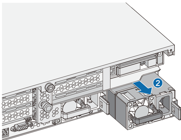
图 2-14 拔出电源模块示意图
