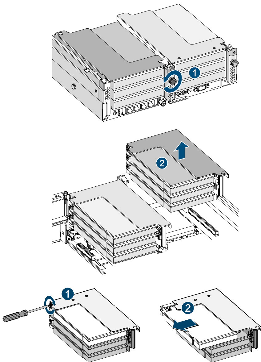
图 2-15 机箱扩展卡安装示意图
