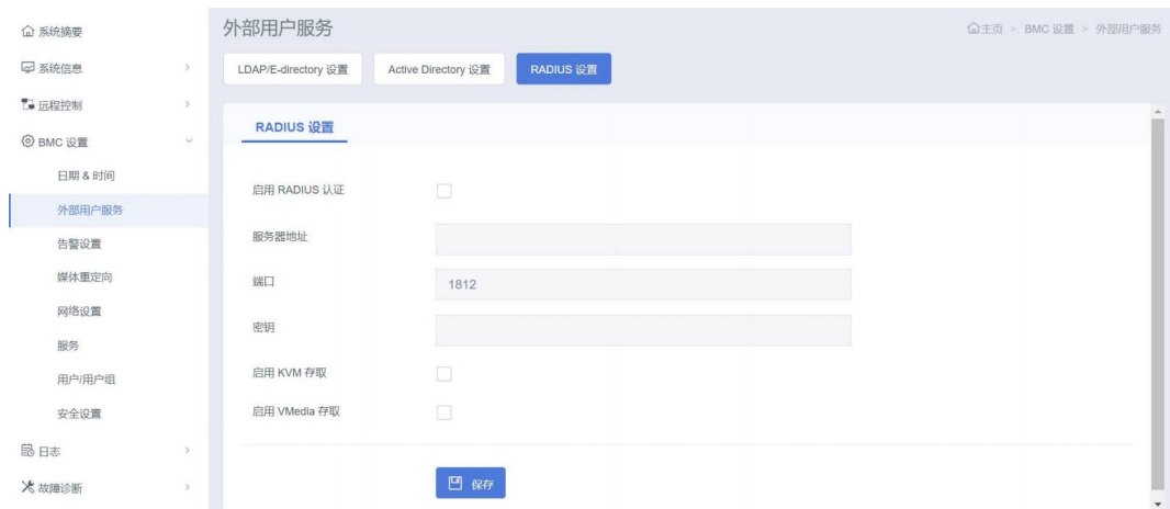
图 3- 87 RADIUS 设置
