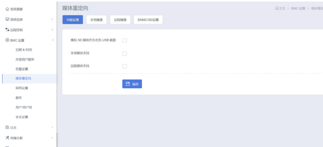
图 3-89 媒体重定向
