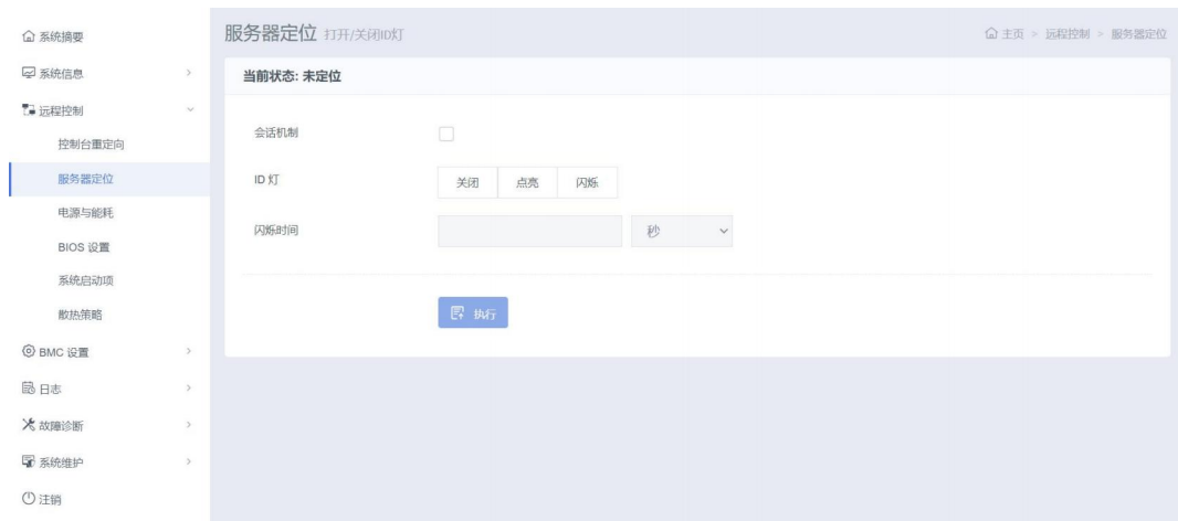
图 3-73 服务器定位
