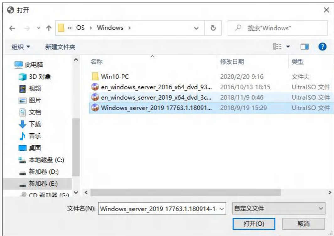
图 4-5 挂载界面
