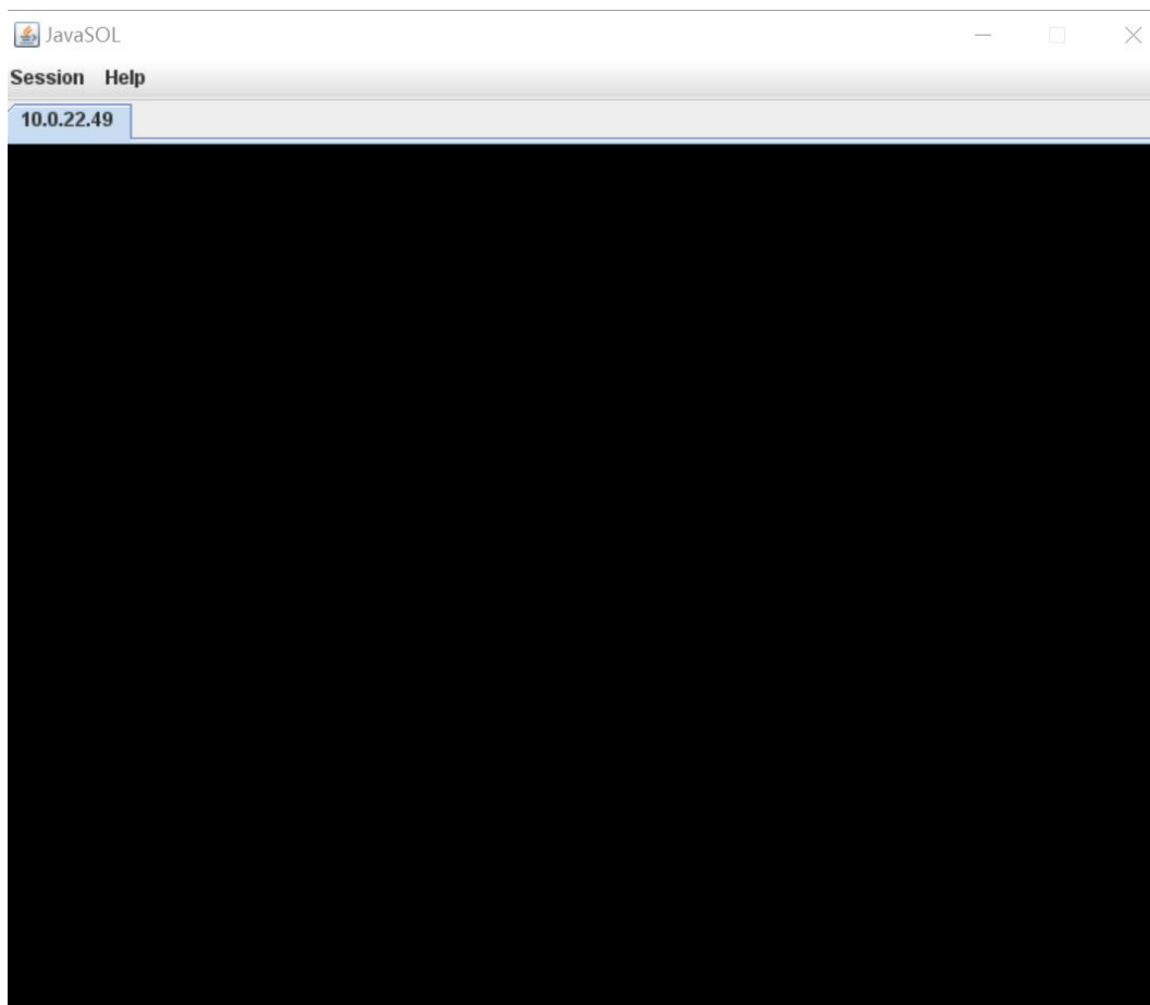
图 3-72 SOL KVM
