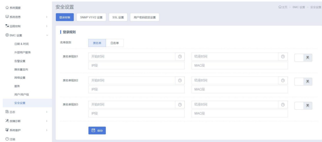
图 3-98 登陆控制
