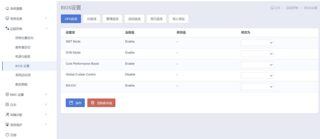
图 3- 80 BIOS 设置
