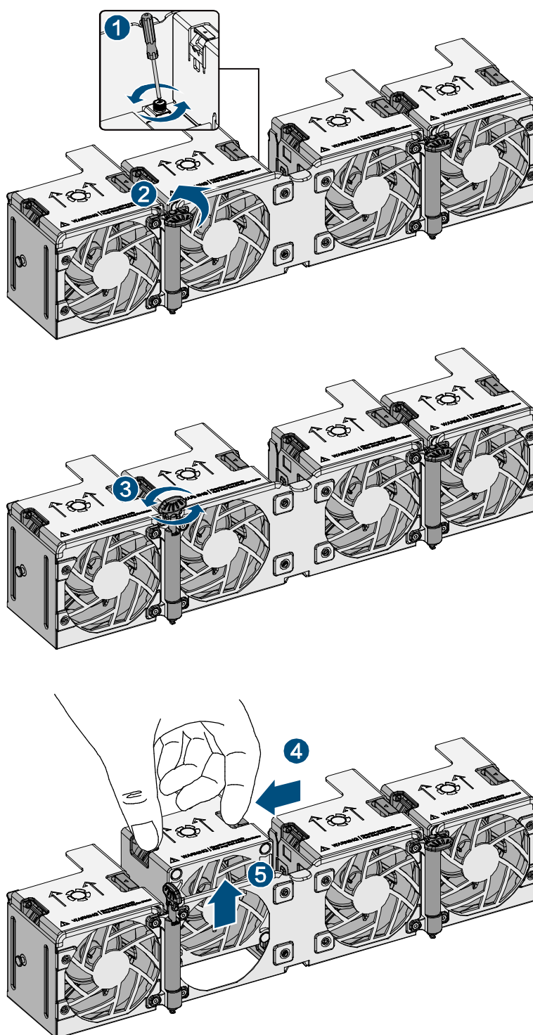
图 2-16 风扇拔出示意图
