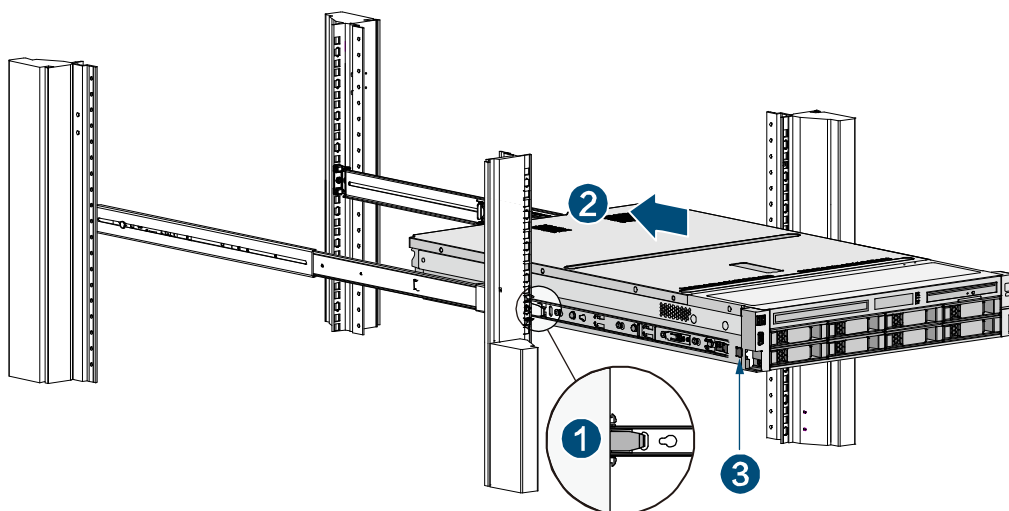
图 2-20 将机器安装到外轨示意图
