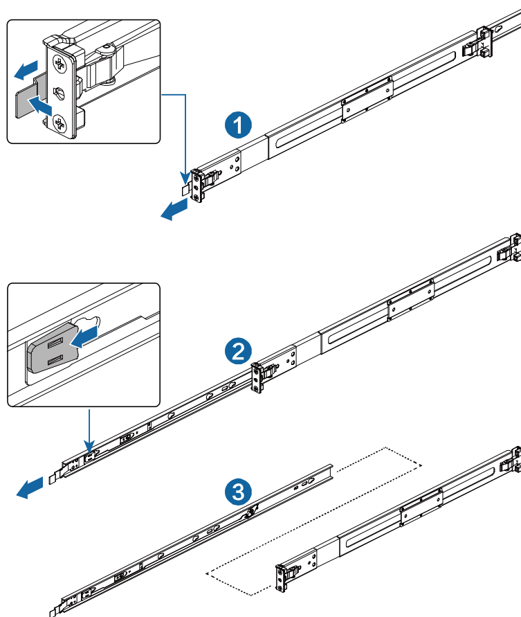
图 2-17 抽出内轨示意图
