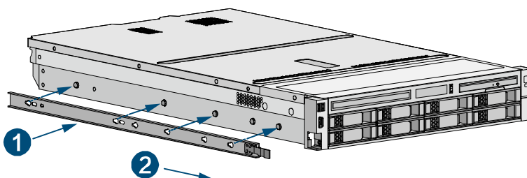
图 2-18 安装内轨示意图
