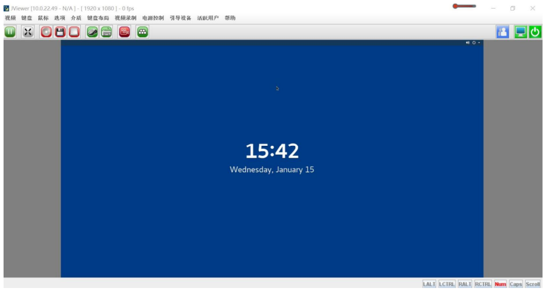
图 3-70 JAVA KVM
