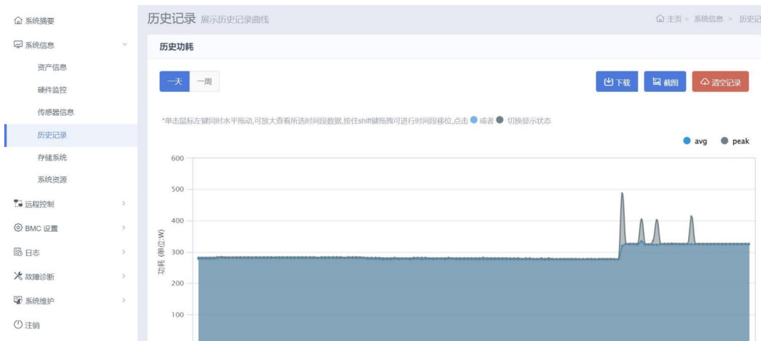
图 3- 65 历史记录
