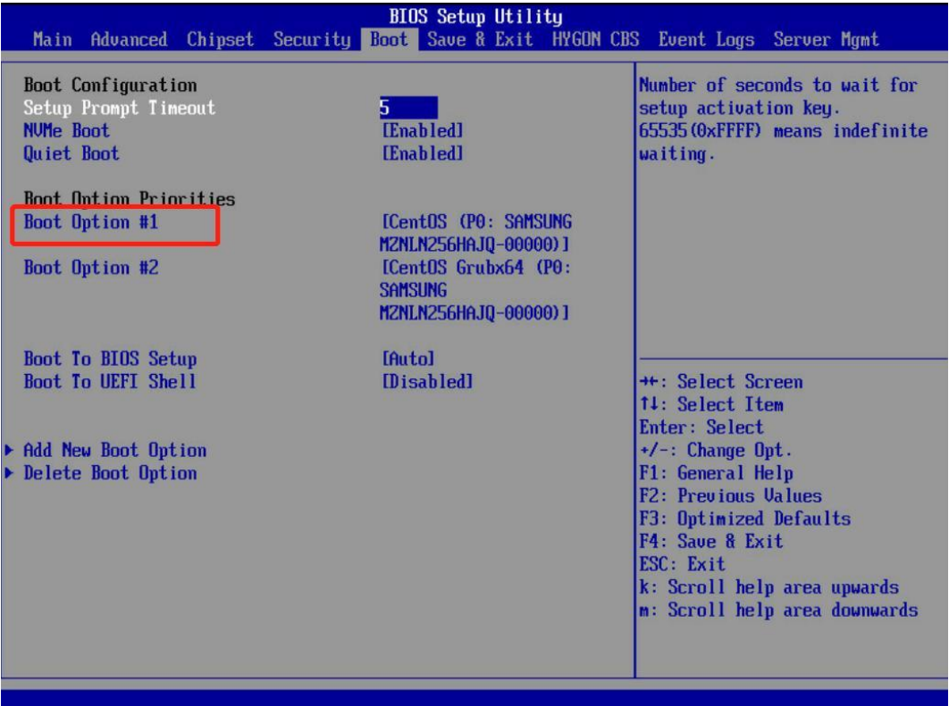
图 4-40 启动项设置
