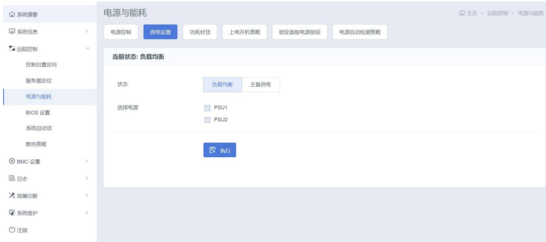
图 3-75 供电设置
