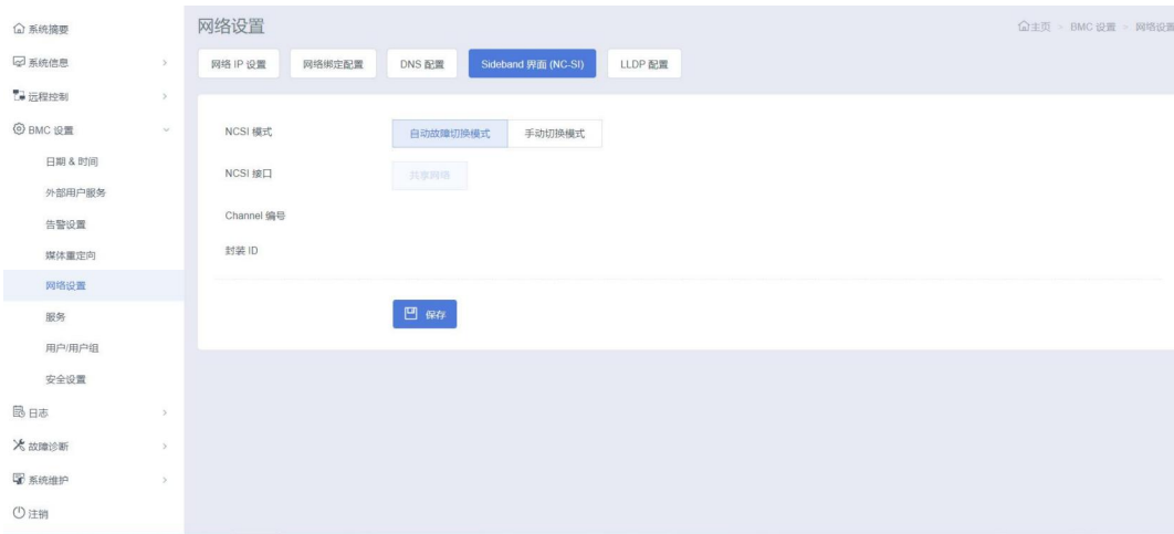
图 3-93 NCSI 配置
