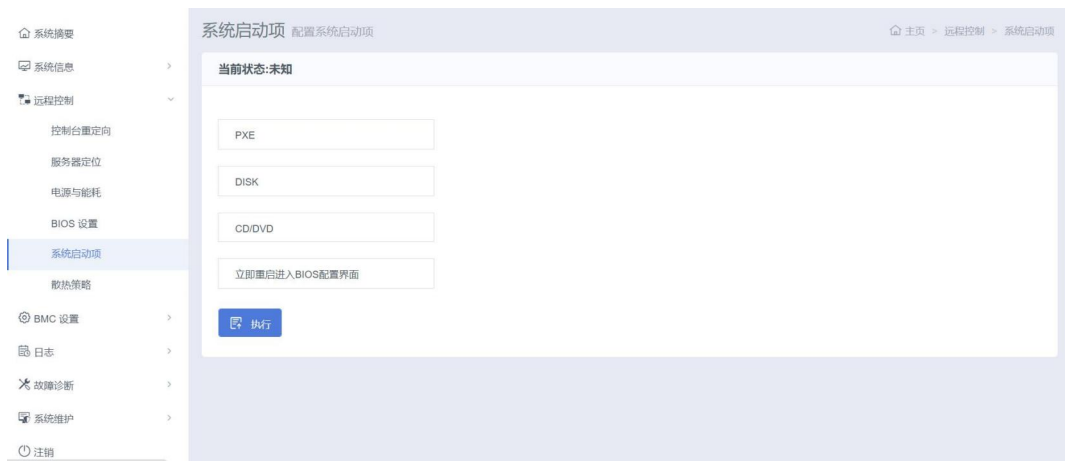
图 3- 81 系统启动项
