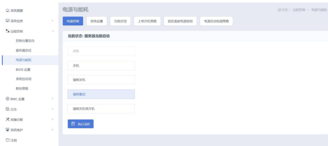
图 3-74 开关机控制
