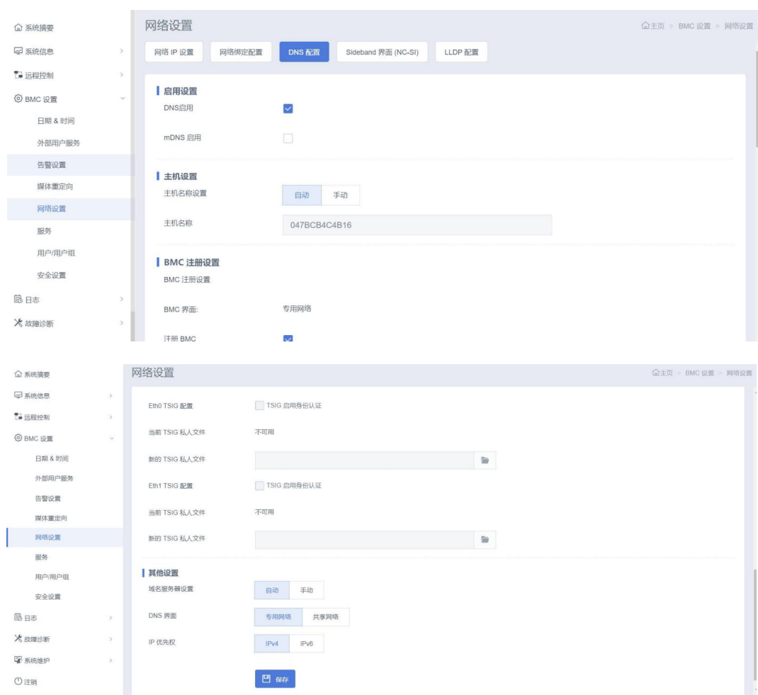
图 3-92 DNS 配置
