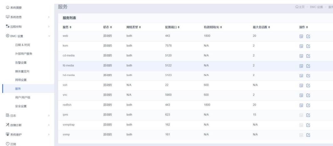
图 3-95 服务设置
