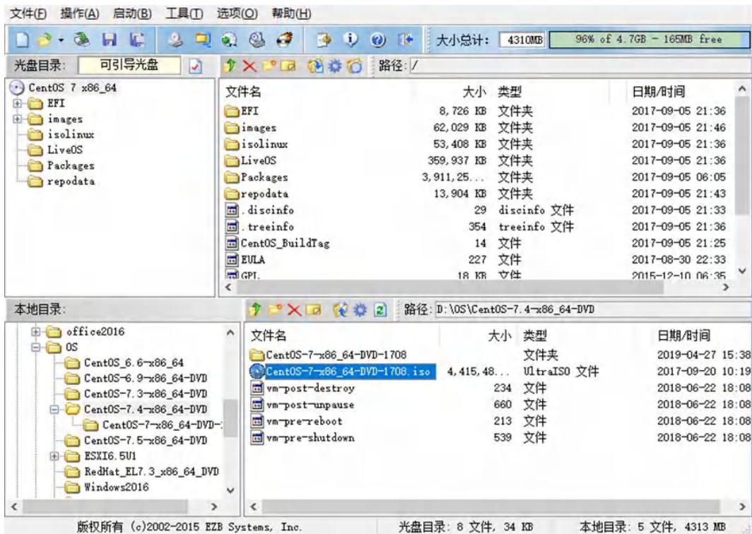
图 4-34 UltraISO 界面
