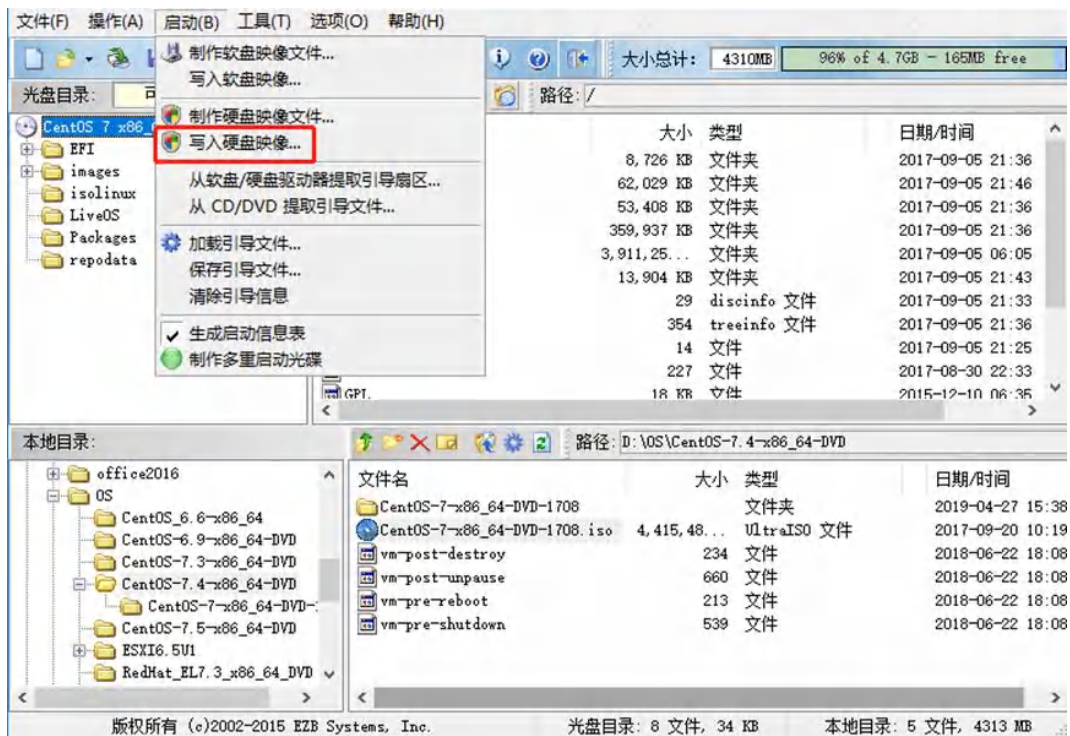
图 4-35 写入镜像
