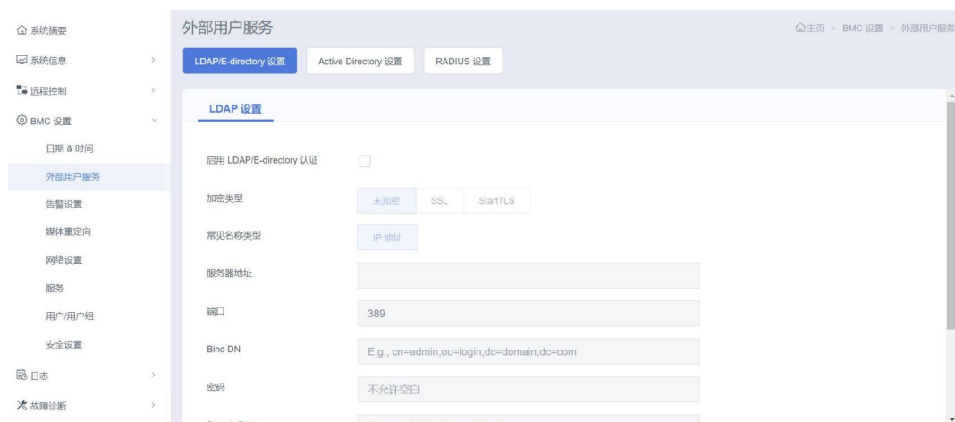
图 3-85 LDAP/E-directory 设置
