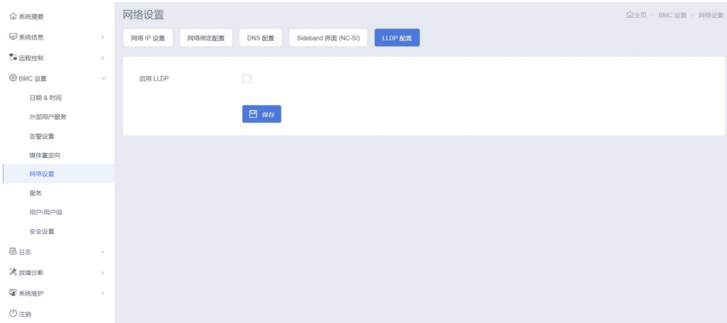
图 3-94 LLDP 配置
