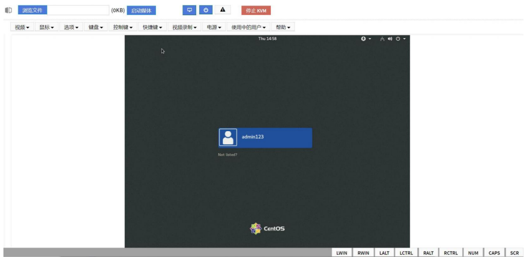
图 3-71 H5 KVM
