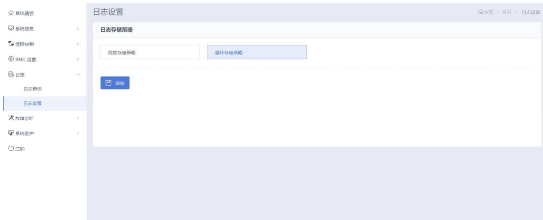
图 3- 106 日志设置
