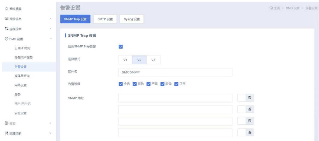
图 3-88 告警设置
