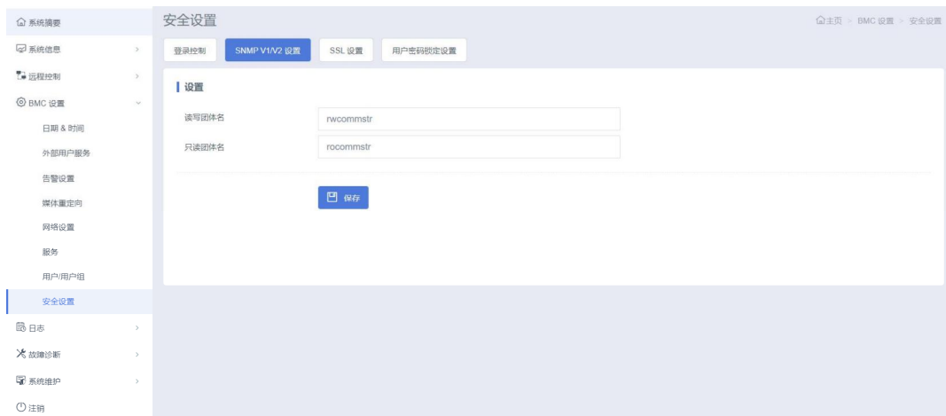
图 3-99 SNMP 设置
