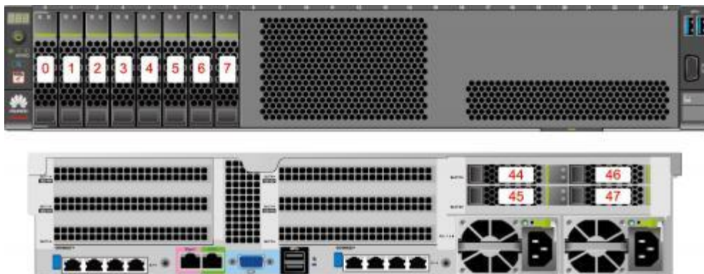
图 7-8 8x2.5 英寸硬盘配置的硬盘编号
