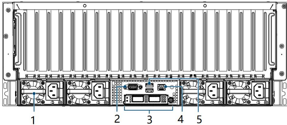
图 2-3 产品后视图
